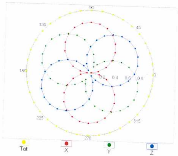
f=1800 MHz,R22
