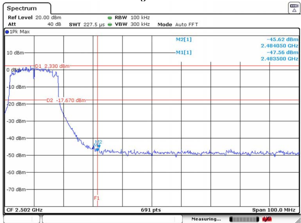
802.11g 2462MHz
