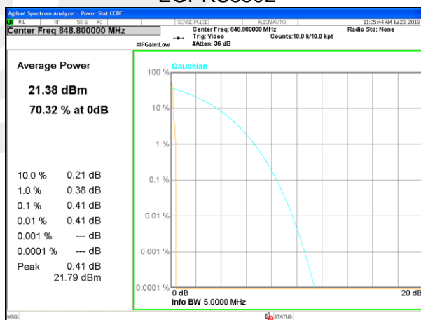
EGPRS850H
