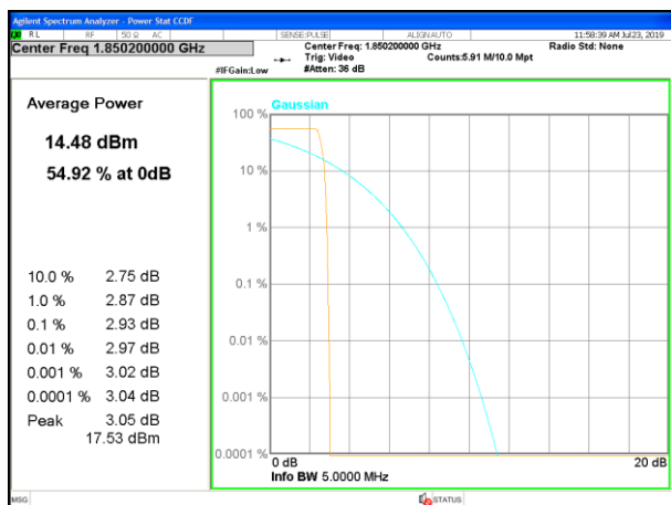
GPRS1900L
