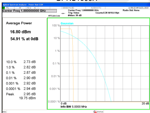
EGPRS1900M
