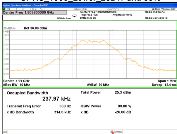
GPRS_1900_Higher_26BW and 99%
