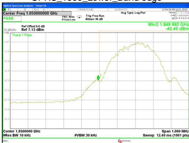
EGPRS_1900_Lower_Band edge
