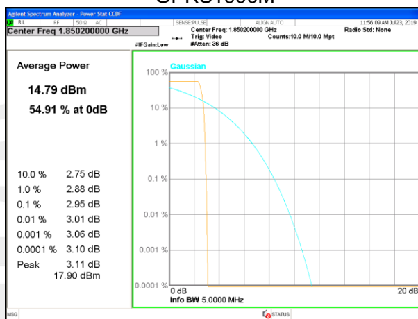
EGPRS1900L
