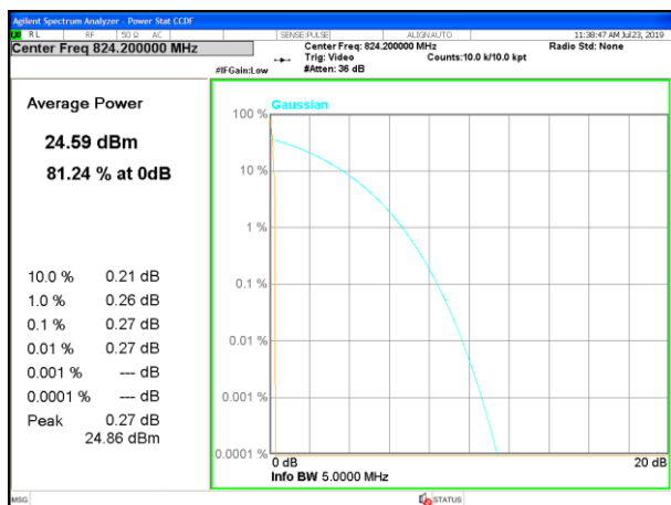
GPRS850L
