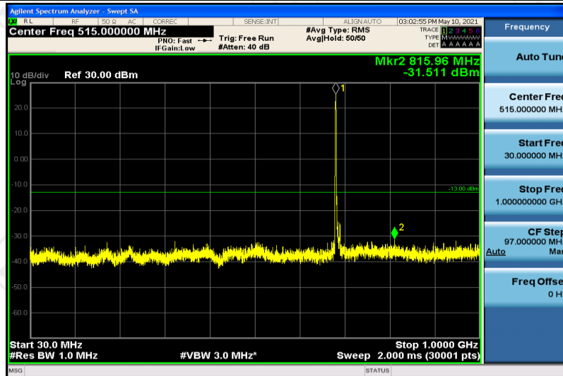
Band71-10MHz-QPSK-133422-1RB#0-Range4:1000~5000MHz
