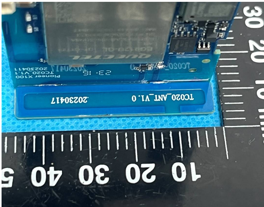
WWAN Antenna
