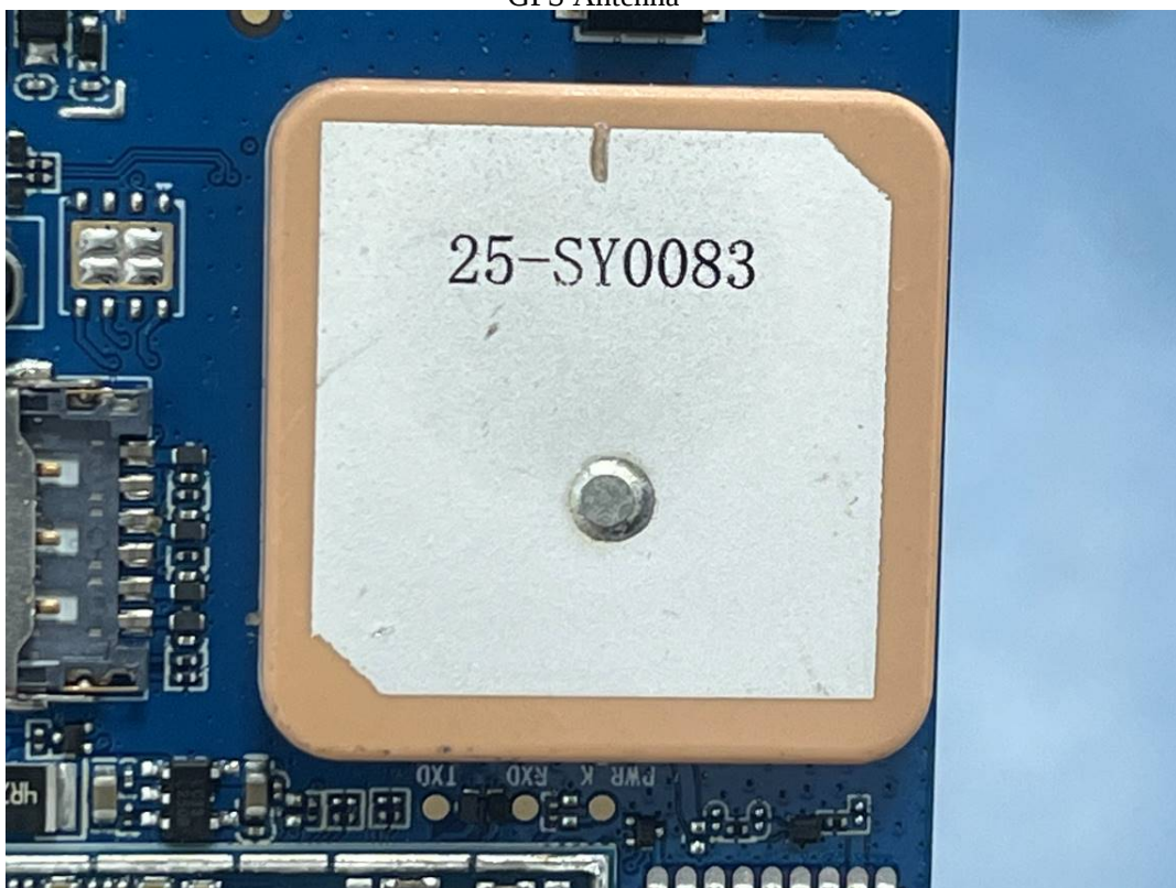
GPS Antenna
