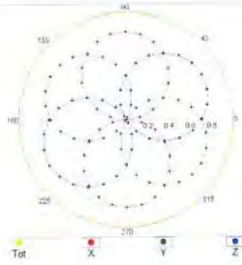
f=1800 MHz,R22
