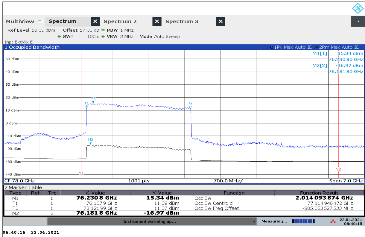
Plot 25: OBW, 10 °C / V nom
