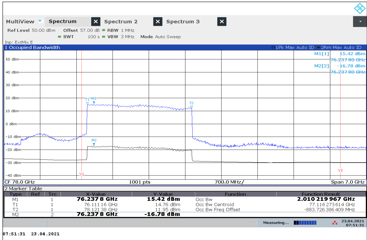
Plot 22: OBW, -20 °C / V nom
