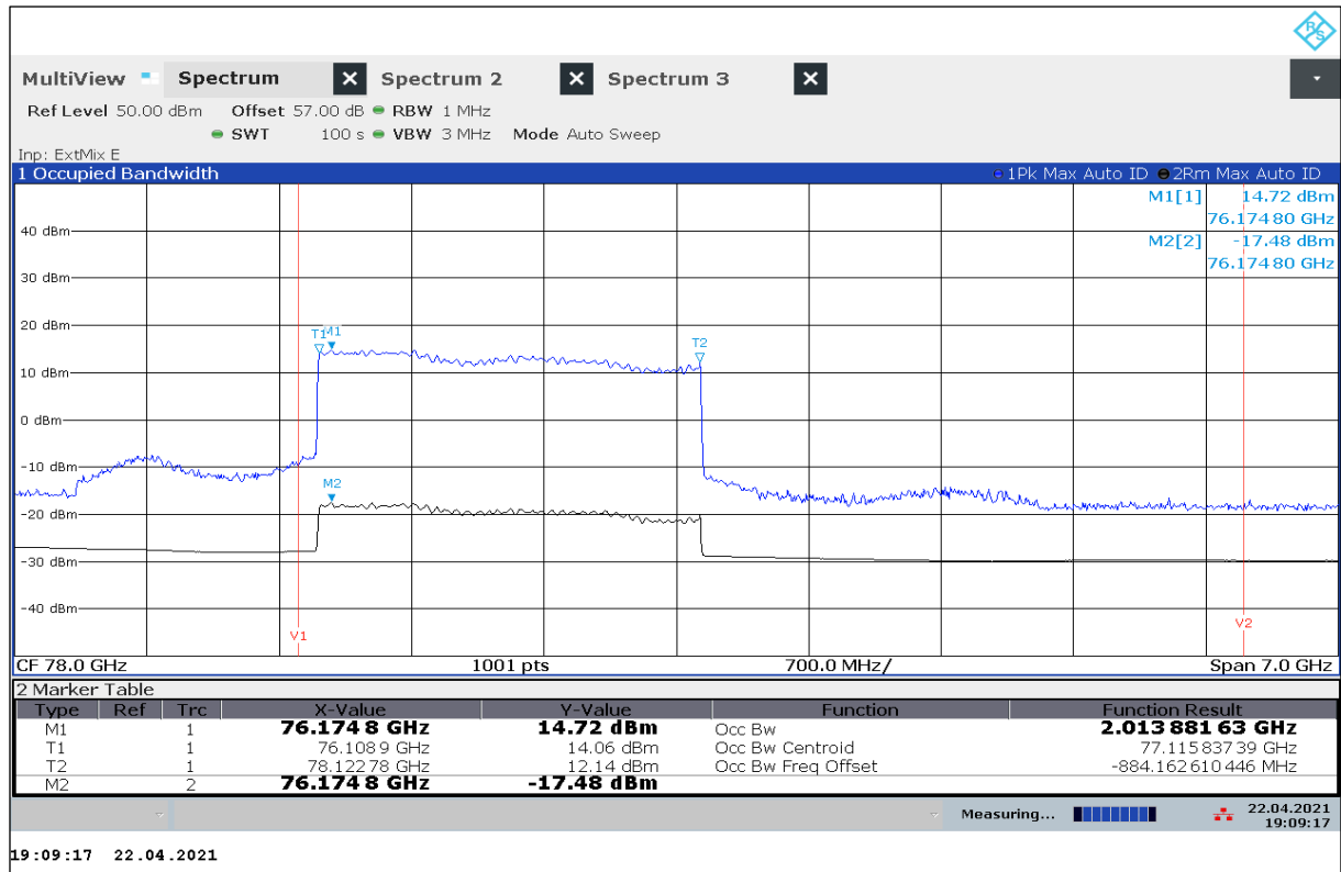
Plot 27: OBW, 30 °C / V nom
