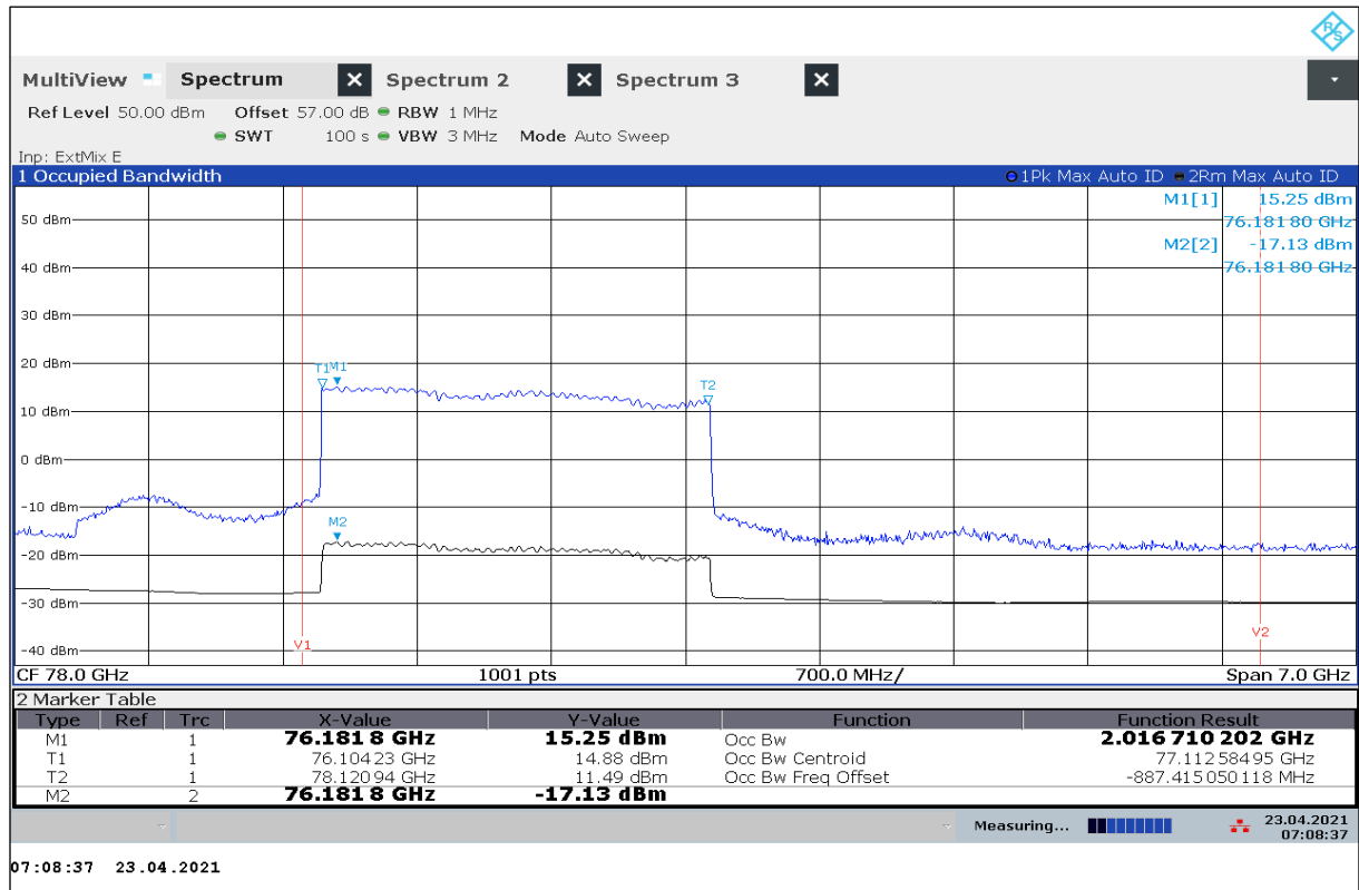
Plot 24: OBW, 0 °C / V nom
