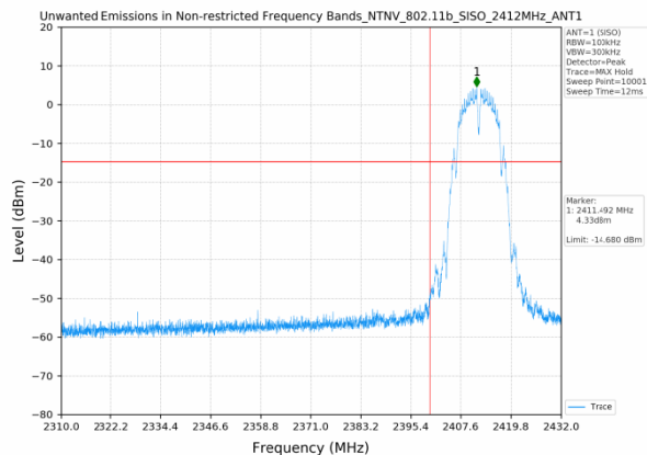
802.11b_2412MHz_SISO ANT1
