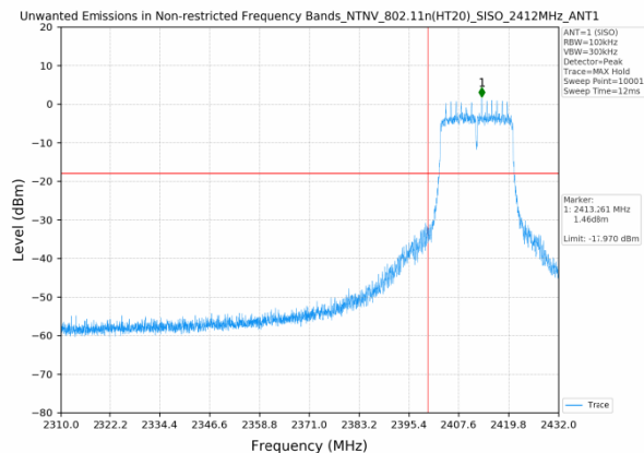
802.11n(HT20)_2412MHz_SISO_ANT1
