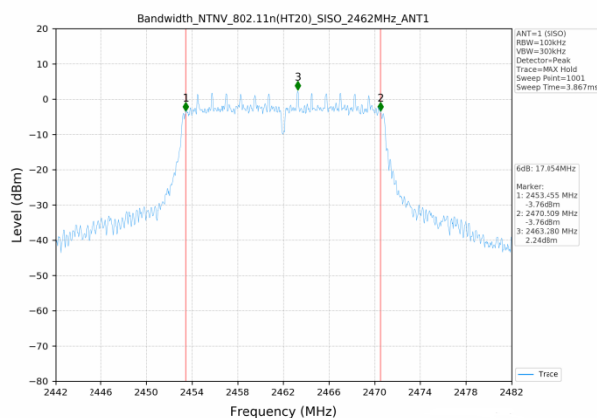
802.11n(HT20) 2462MHz SISO ANT1
