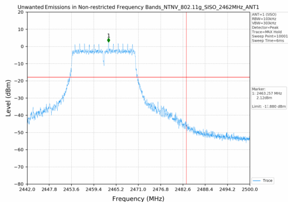
802.11g_2462MHz_SISO_ANT1
