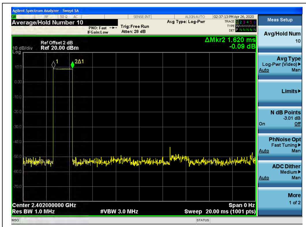
(DH3, GFSK)
