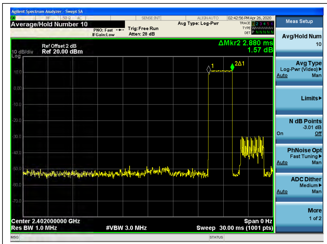
(DH5, 8-DPSK)
