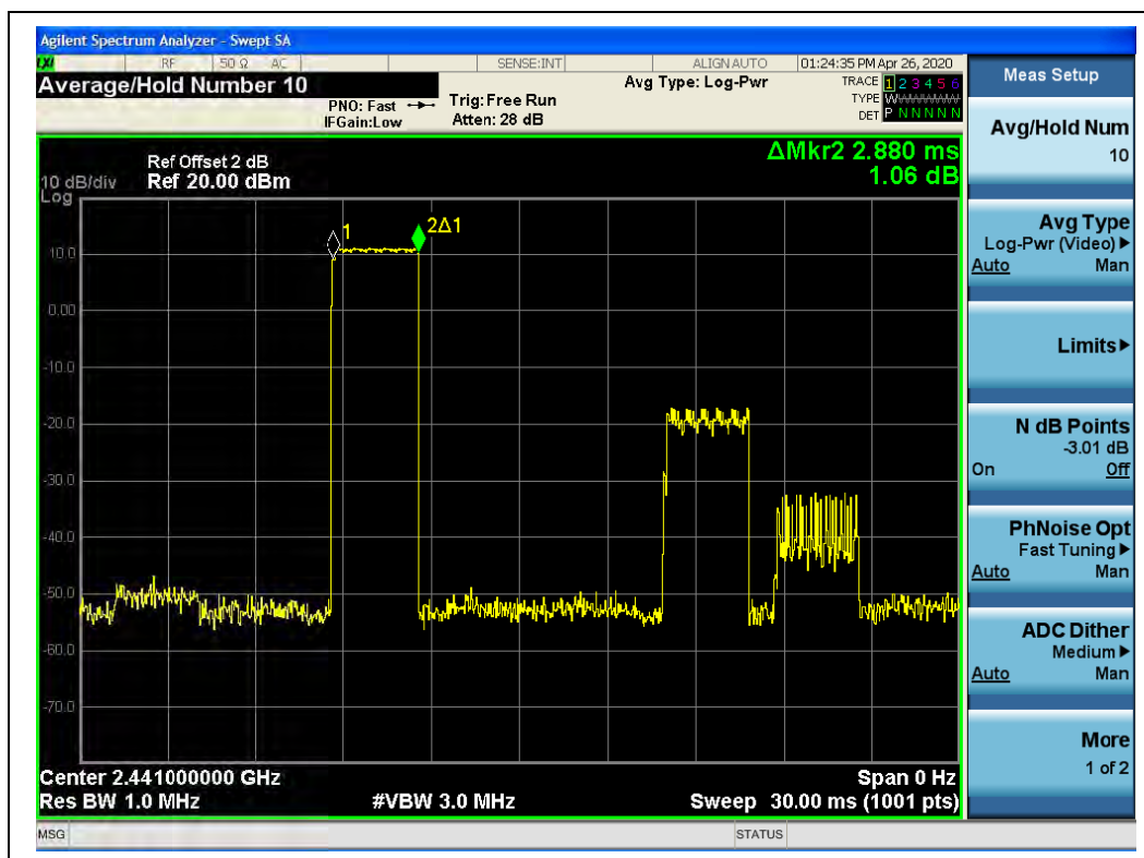
(DH5, 8-DPSK)
