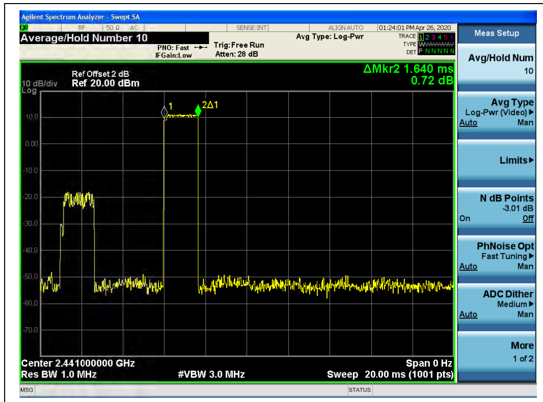
(DH3, 8-DPSK)
