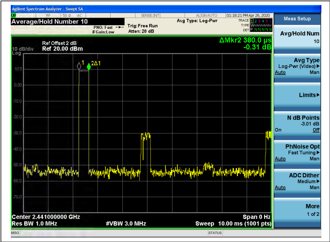
(DH1, GFSK)
