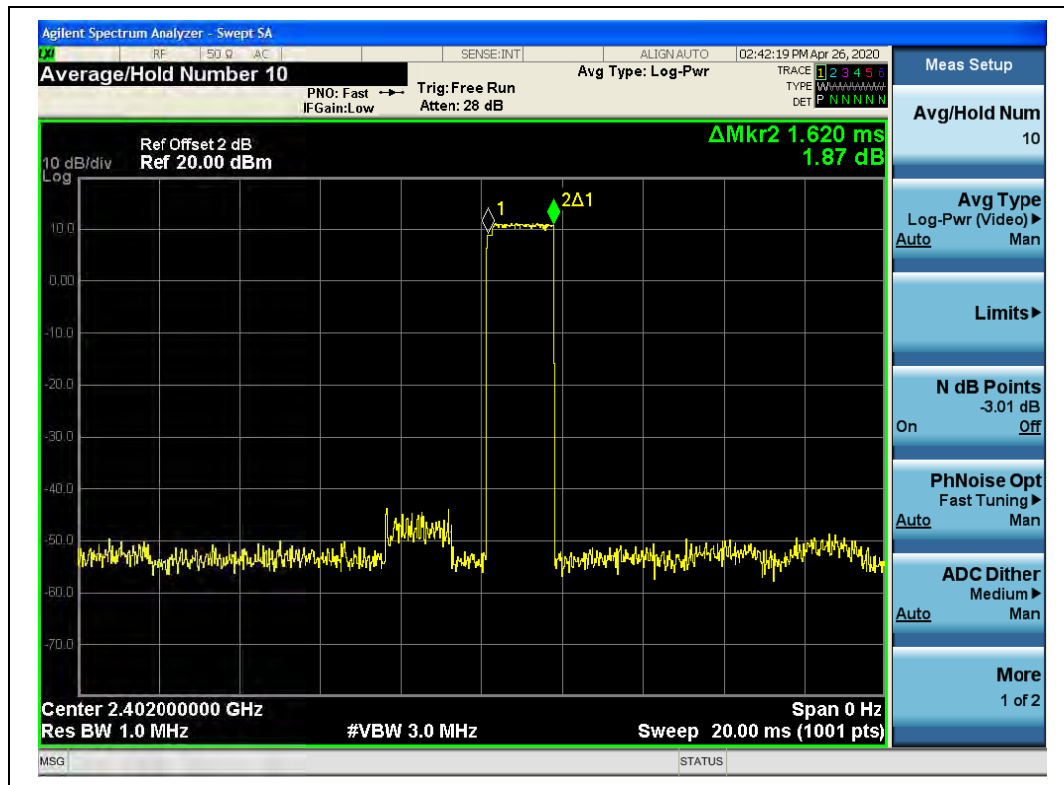
(DH3, 8-DPSK)
