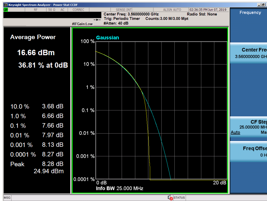
LTE Band 48 / 20 MHz / QPSK
