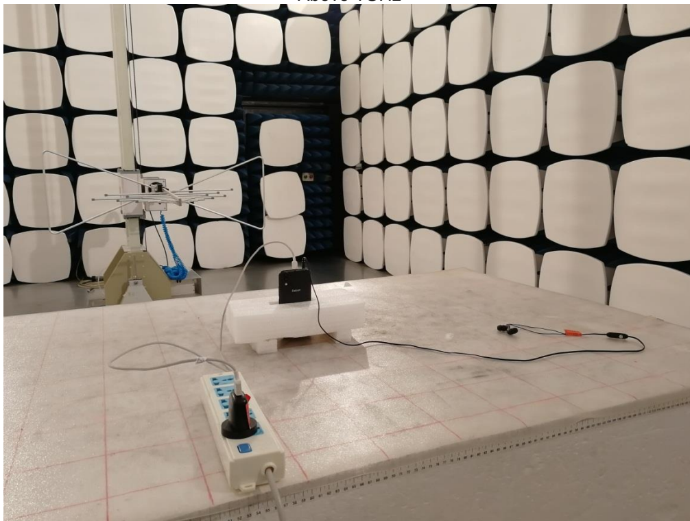
AU Above 1GHz
