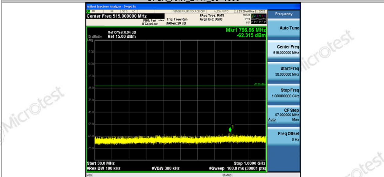
GFSK_Ant1_2441_30~1000
