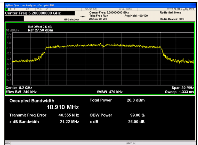
IEEE 802.11ax_Channel 40_20MHz_Antenna 1_RU&Index SU
