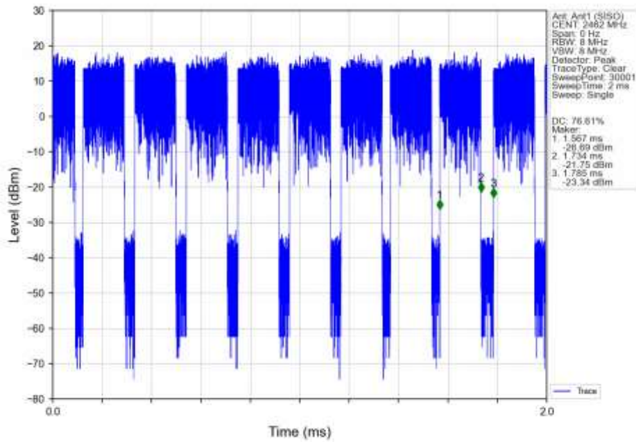
802.11n(HT20)_HCH_2462MHz_Ant1 (SISO)_NTNV
