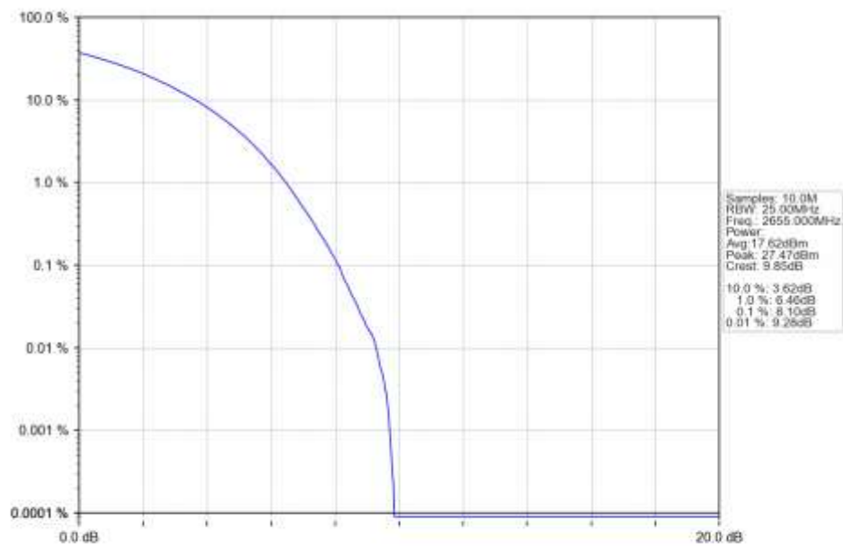
n41_30kHz_SISO_NTNV_70MHz_CP-OFDM_16_QAM_2655MHz_Outer_Full_Ant1
