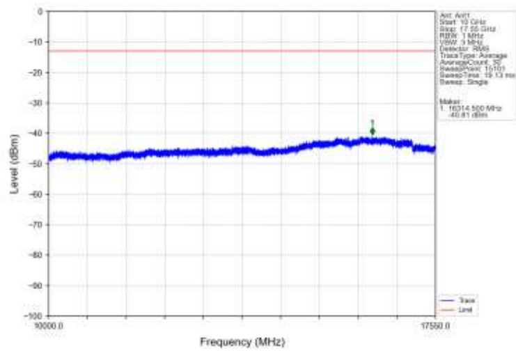
Band4_HSUPA_LCH_1712.4MHz_Subtest 1_NTNV
