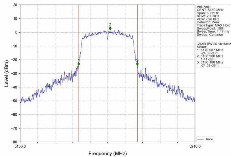
802.11ac(VHT20) LCH_5180MHz_Ant1_NTNV
