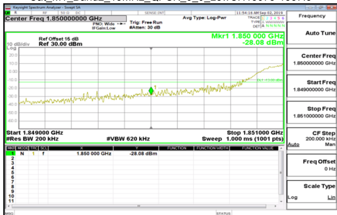
Cat_M1_Band2_15MHz_QPSK_6_0_LowCH18675-1857.5
