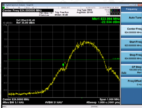
GSM 850-LCH-GPRS
