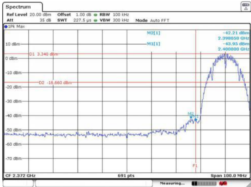
IEEE 802.11b 2412MHz
