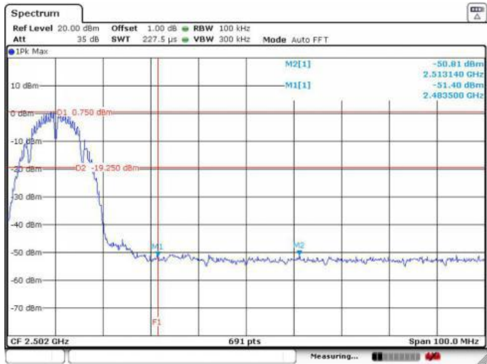
IEEE 802.11b 2462MHz
