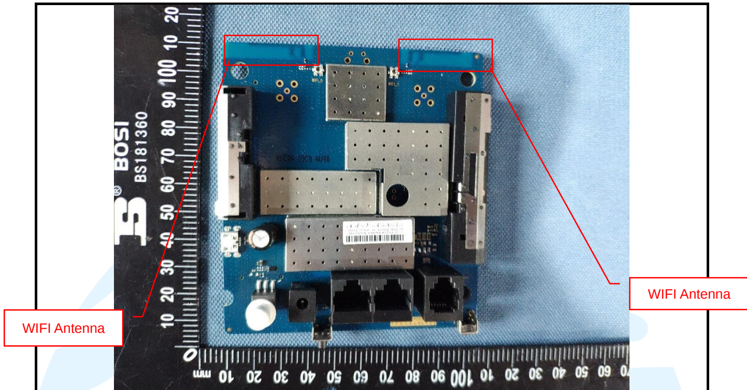
EUT Photo
