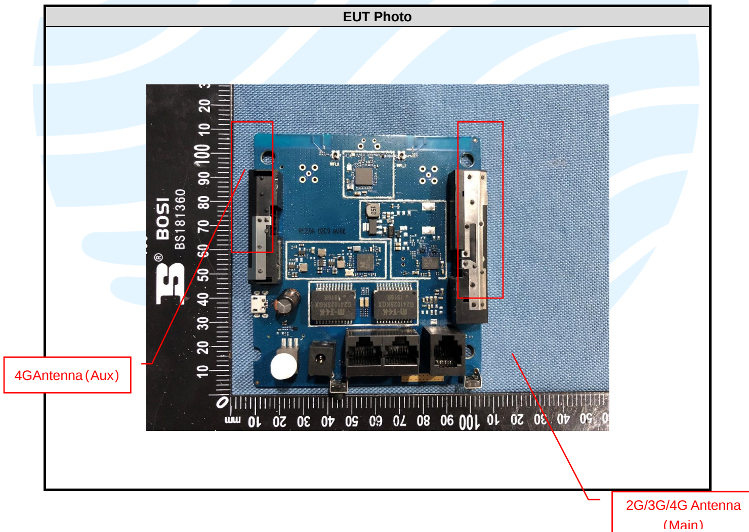
EUT Photo
