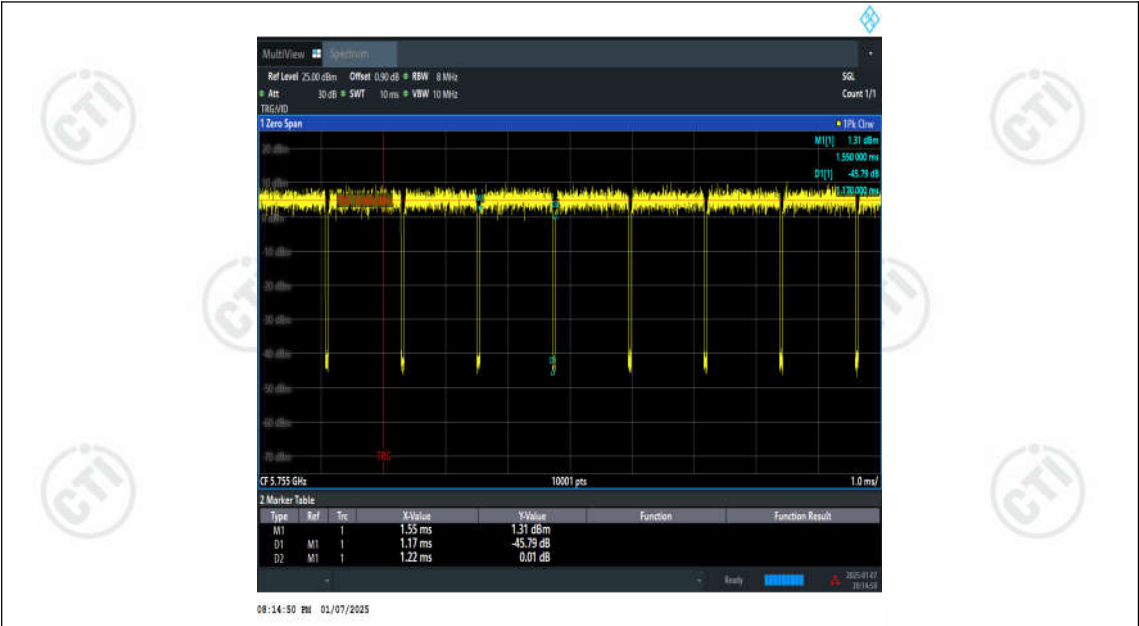
NTNV-11AX40ISO-Ant1-5755
