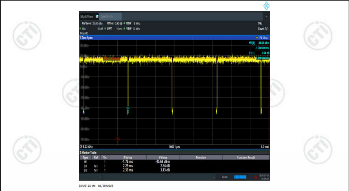
NTNV-11AX20MIMO-Ant1-5220
