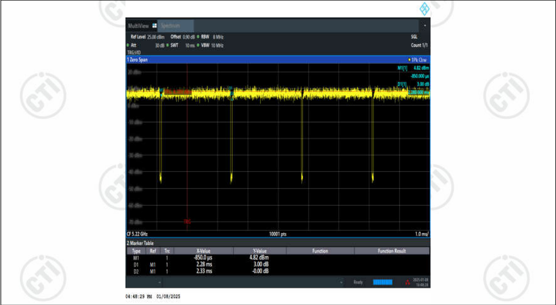
NTNV-11AX20MIMO-Ant2-5220
