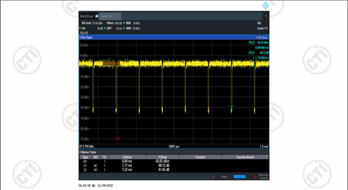
NTNV-11AX40MIMO-Ant2-5795
