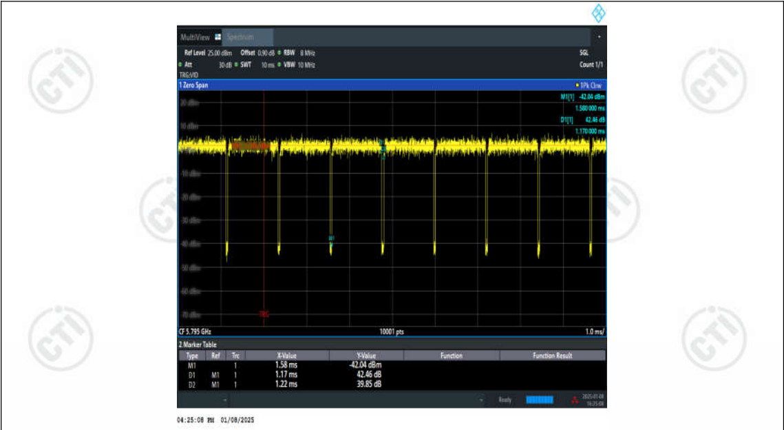
NTNV-11AX40MIMO-Ant1-5795
