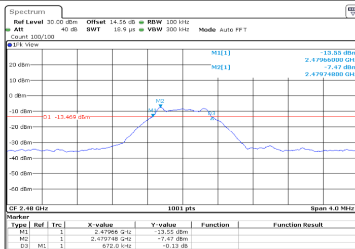
BLE_Ant1_2480
