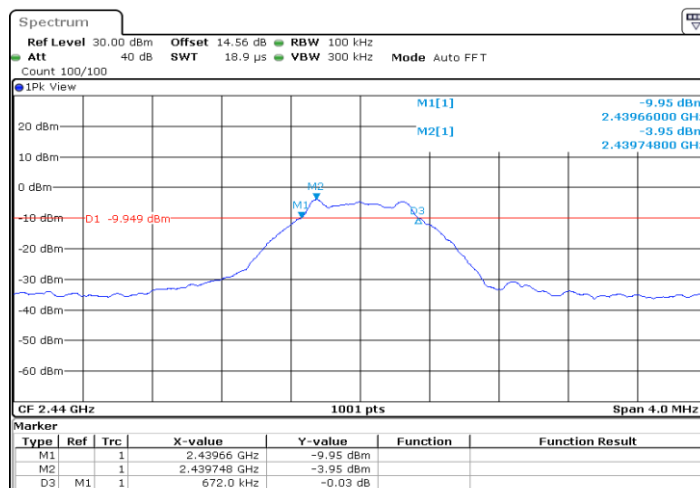
BLE_Ant1_2440
