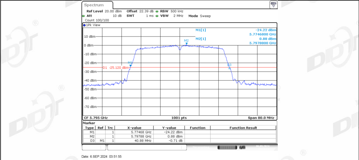
11N40MIMO_Ant2_5795
