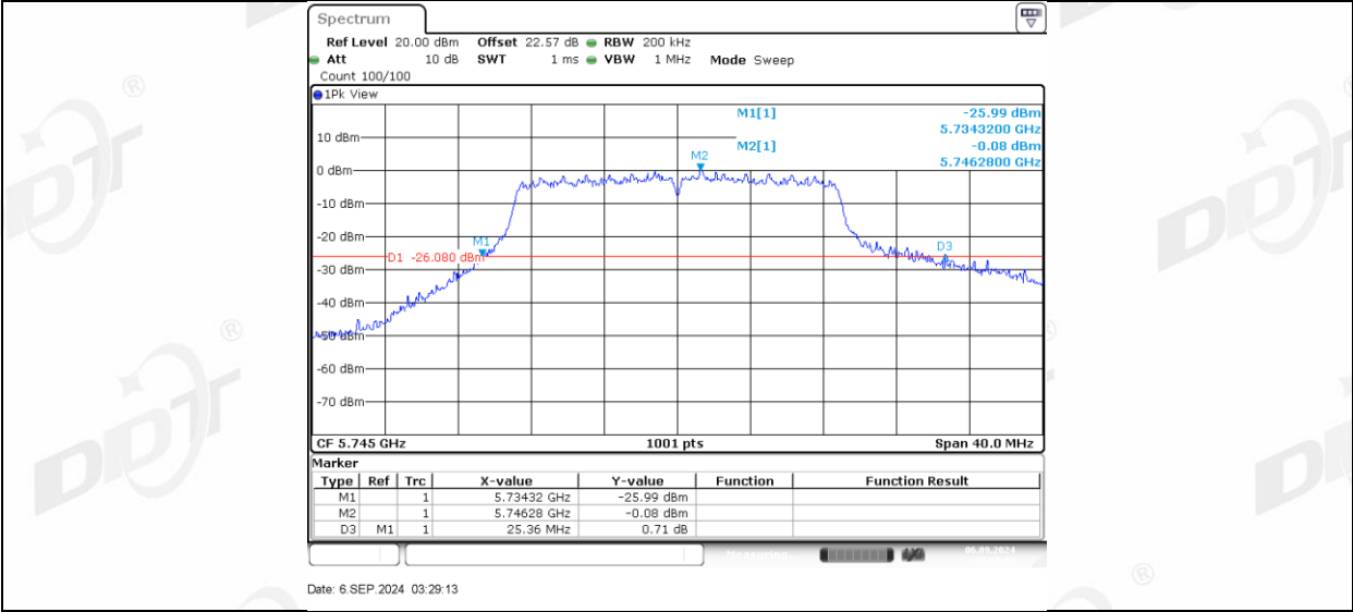
11N20MIMO_Ant2_5745
