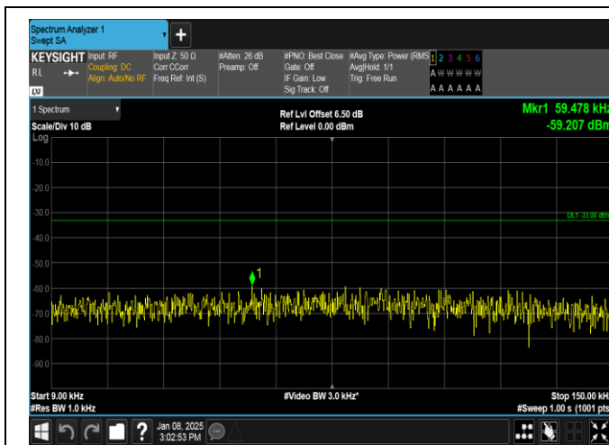
Band26(824-849)-3MHz-QPSK-27025-1RB#0-0.009~0.15-PASS
