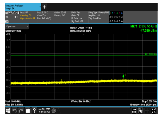
Band26(824-849)-3MHz-QPSK-27025-1RB#0-1000~3000-PASS
