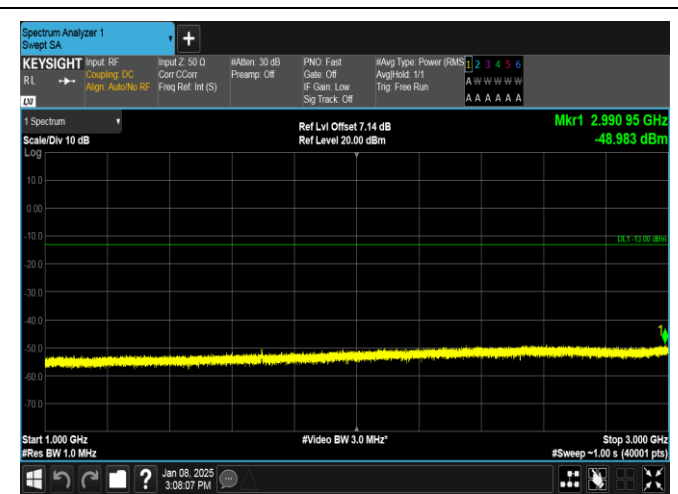
Band26(824-849)-3MHz-QPSK-27025-15RB#0-1000~3000-PASS
