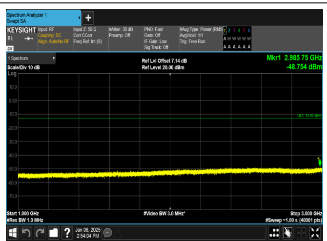
Band26(824-849)-3MHz-QPSK-26805-15RB#0-1000~3000-PASS
