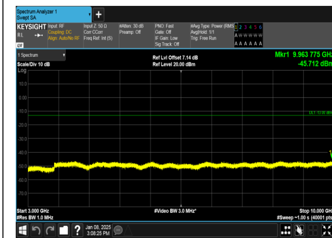
Band26(824-849)-3MHz-QPSK-27025-15RB#0-3000~10000-PASS
