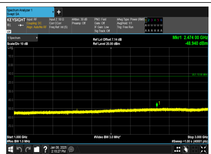
Band26(824-849)-1.4MHz-QPSK-26797-6RB#0-1000~3000-PASS
