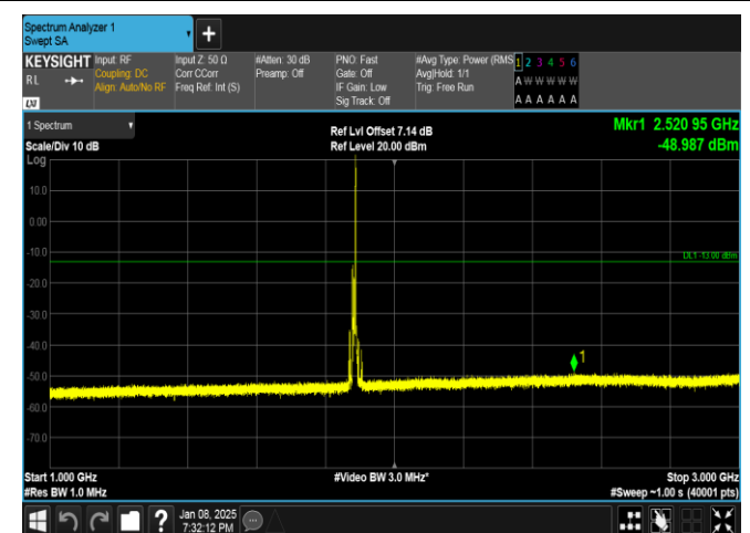
Band25-10MHz-QPSK-26365-1RB#49-1000~3000-PASS
