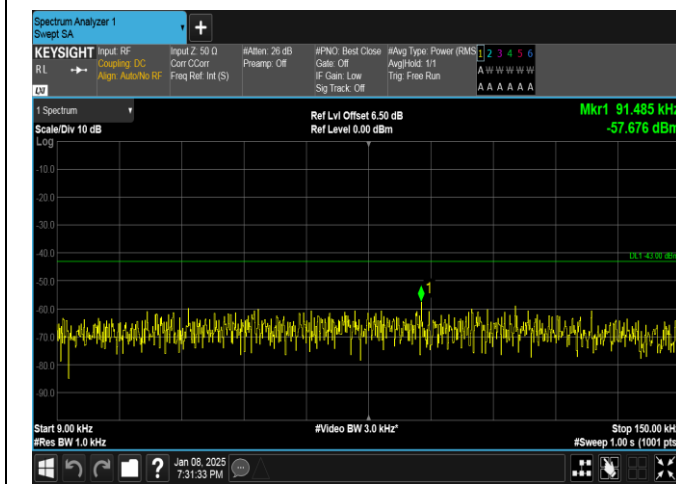
Band25-10MHz-QPSK-26365-1RB#49-0.009~0.15-PASS
