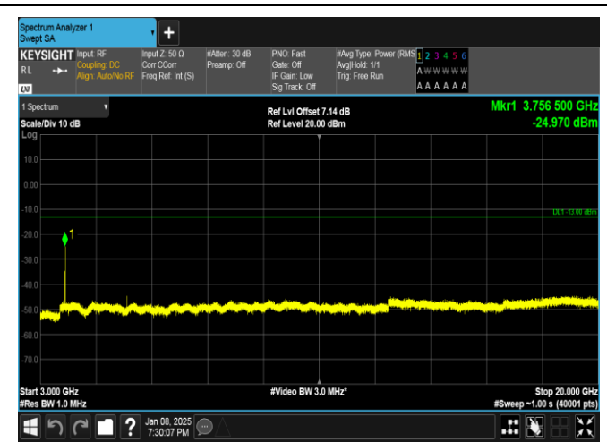
Band25-10MHz-QPSK-26365-1RB#0-3000~20000-PASS
