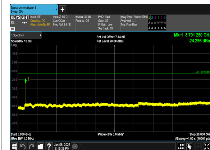
Band25-15MHz-QPSK-26115-1RB#0-3000~20000-PASS
