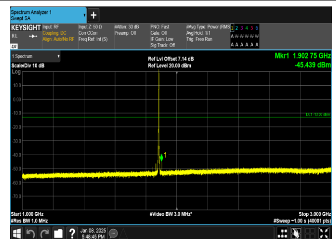
Band25-3MHz-QPSK-26365-1RB#14-1000~3000-PASS
