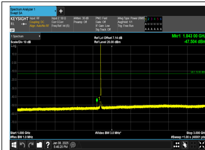
Band25-3MHz-QPSK-26365-1RB#0-1000~3000-PASS
