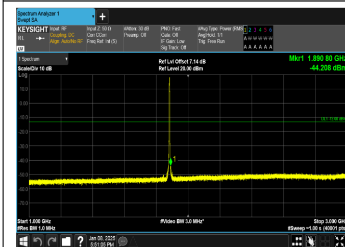
Band25-3MHz-QPSK-26365-15RB#0-1000~3000-PASS
