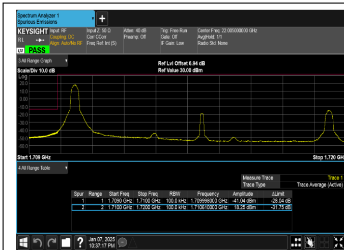
Band4-10MHz-QPSK-20000-1RB#0-PASS
