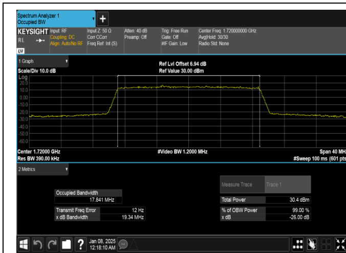
Band4-20MHz-QPSK-20050-100RB#0-PASS
