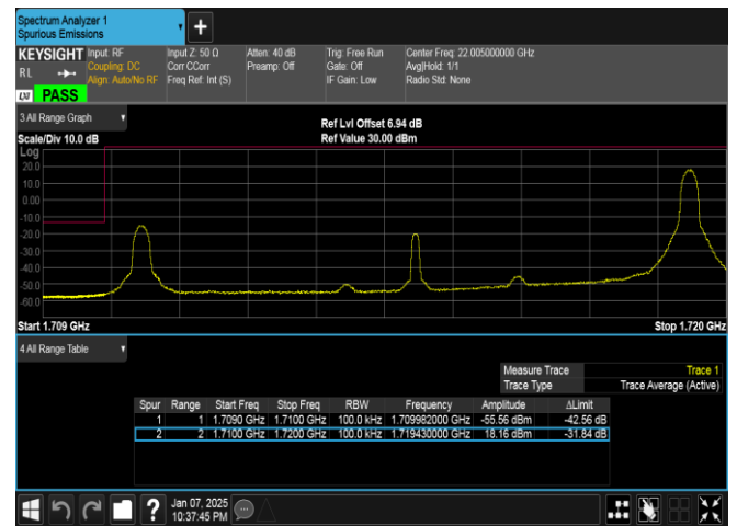
Band4-10MHz-QPSK-20000-1RB#49-PASS
