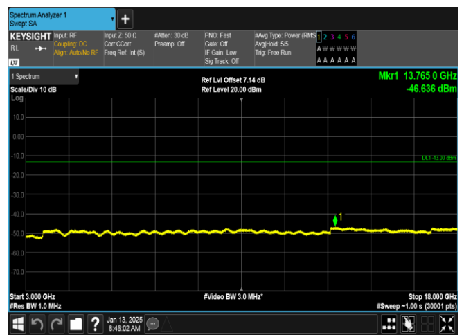
GPRS1900-810-0-3000~18000MHz-PASS
