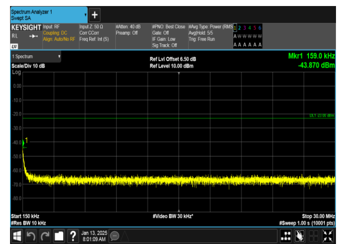
GPRS850-251-5-0.15~30MHz-PASS
