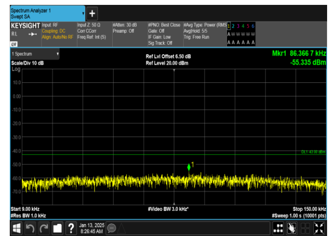
GSM1900-661-0-0.009~0.15MHz-PASS
