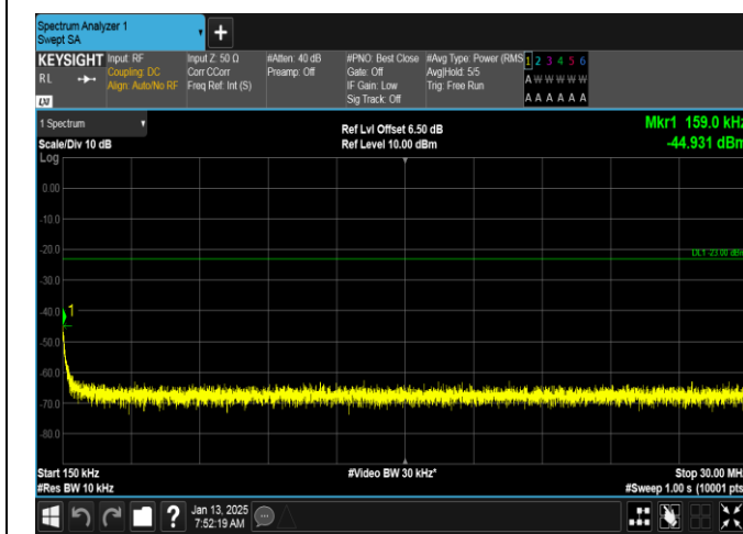
GSM850-251-5-0.15~30MHz-PASS
