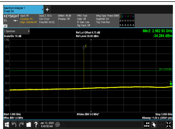
GPRS1900-810-0-1000~3000MHz-PASS
