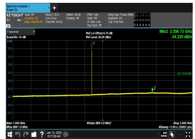
GSM1900-661-0-1000~3000MHz-PASS
