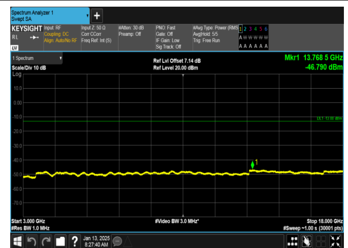
GSM1900-661-0-3000~18000MHz-PASS
