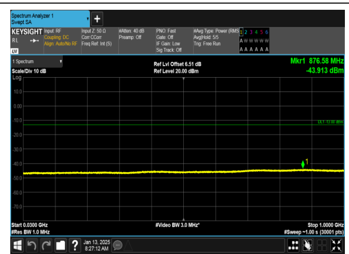
GSM1900-661-0-30~1000MHz-PASS
