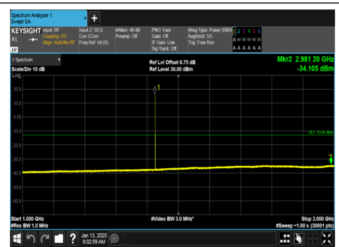
EGPRS1900-512-2-1000~3000MHz-PASS
