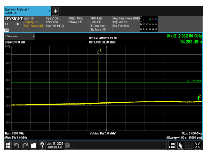
EGPRS1900-810-2-1000~3000MHz-PASS
