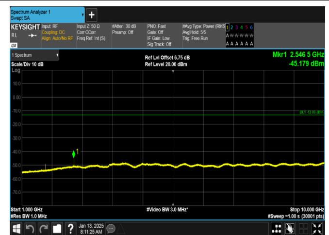
EGPRS850-251-8-1000~10000MHz-PASS
