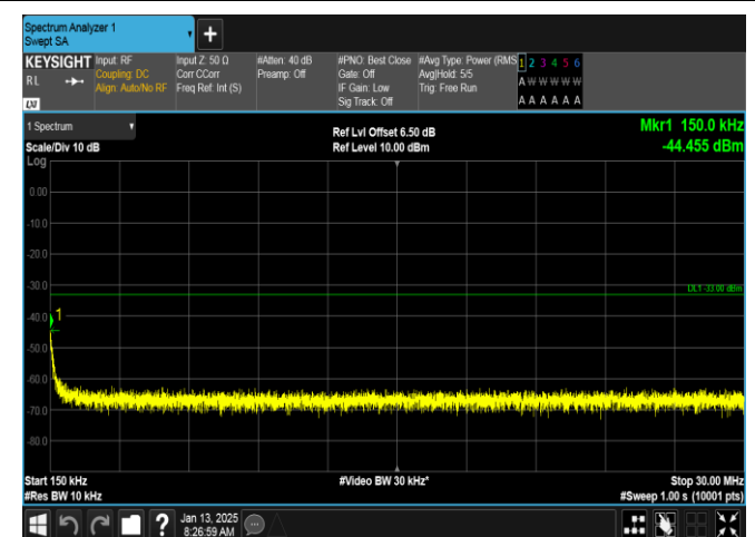
GSM1900-661-0-0.15~30MHz-PASS
