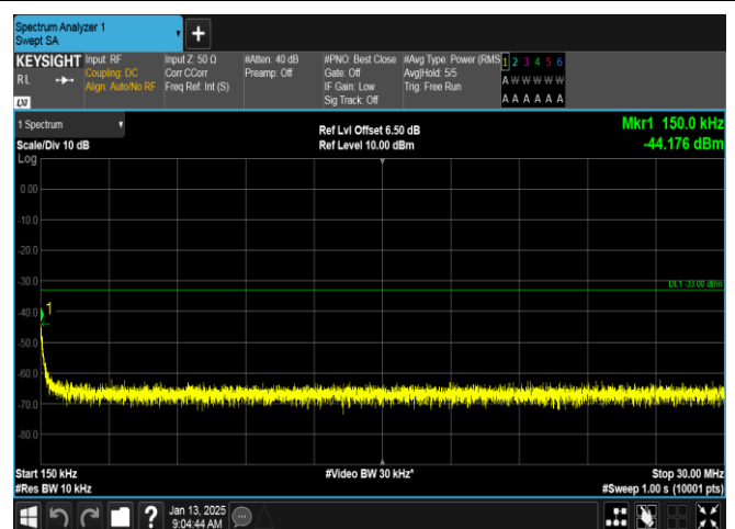
EGPRS1900-810-2-0.15~30MHz-PASS
