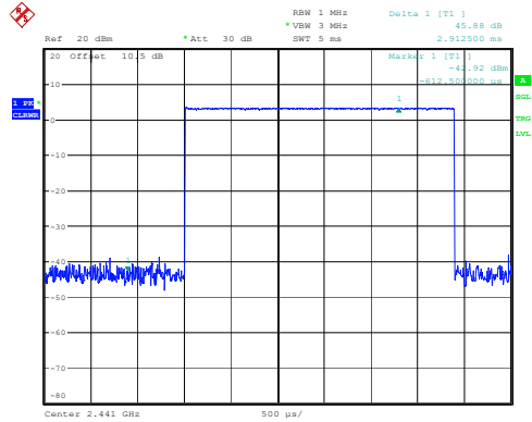
DH5_Hopping 2.913ms
