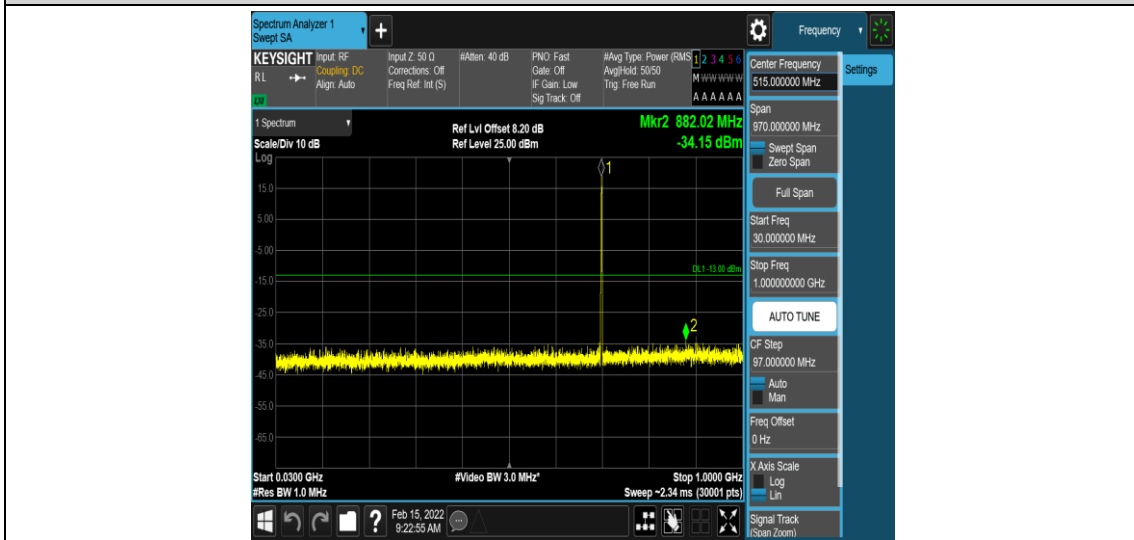
Band12-3MHz-QPSK-23095-1-0-Low-30-1000--34.15-PASS
