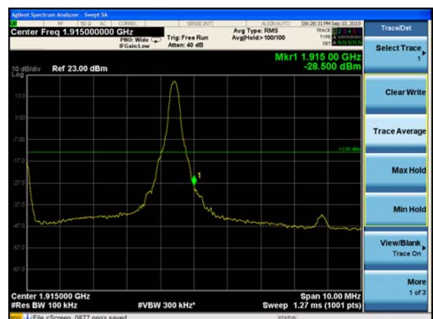
LTE Band 25 10MHz QPSK 1RB CH-High
