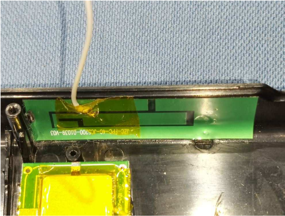
LTE Antenna
