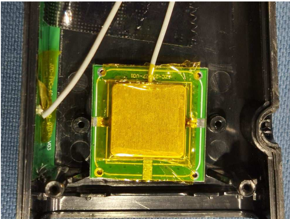
GPS Antenna
