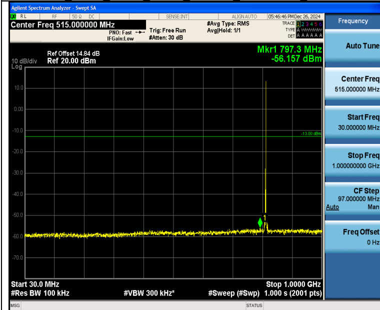
Band26 3MHz QPSK 26705 1RB#14 30~1000 30~1000
