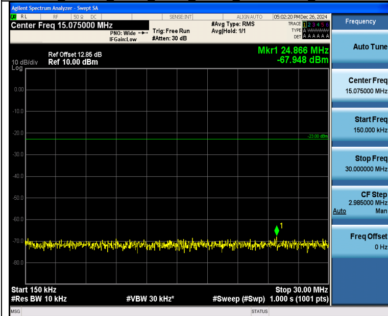
Band26 1.4MHz 16QAM 26740 6RB#0 0.15~30 0.15~30
