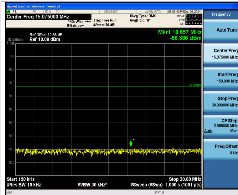
Band26 1.4MHz 16QAM 26783 1RB#5 0.15~30 0.15~30
