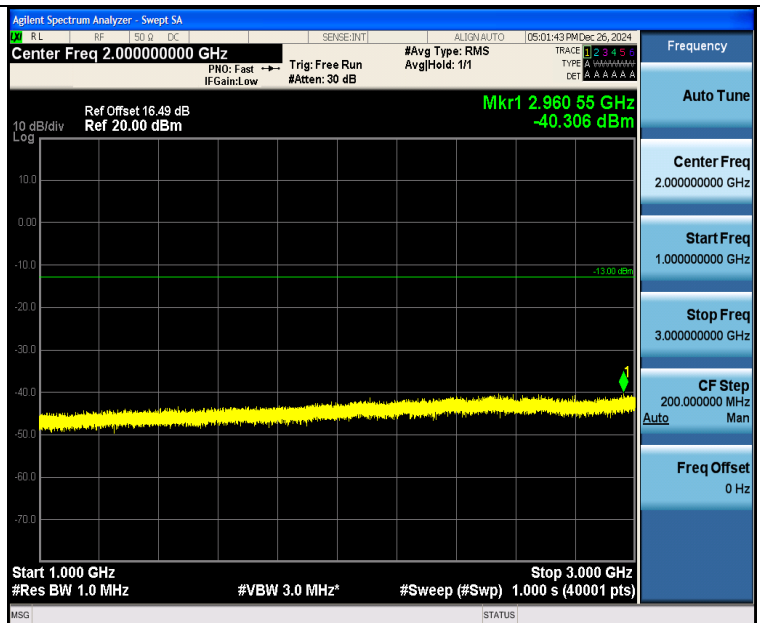
Band26 1.4MHz QPSK 26740 6RB#0 1000~3000 1000~3000
