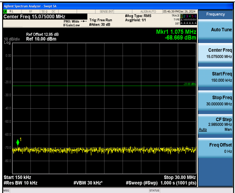
Band26 3MHz QPSK 26705 1RB#14 0.15~30 0.15~30
