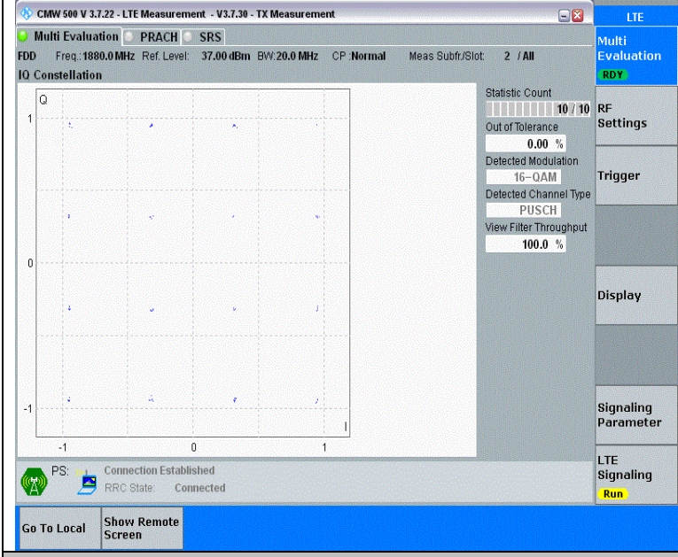
Band2-20MHz-16QAM-18900-1RB#0-PASS
