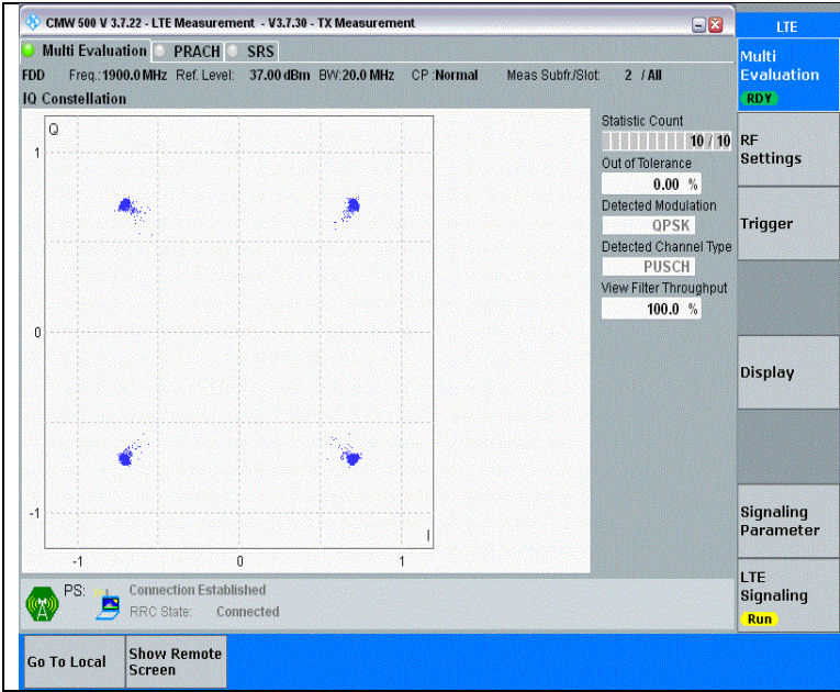
Band2-20MHz-QPSK-19100-100RB#0-PASS
