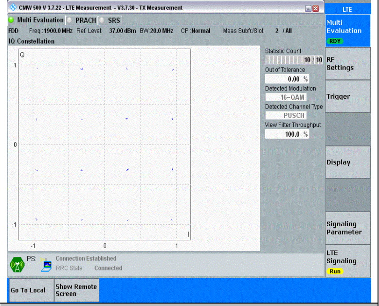
Band2-20MHz-16QAM-19100-1RB#0-PASS
