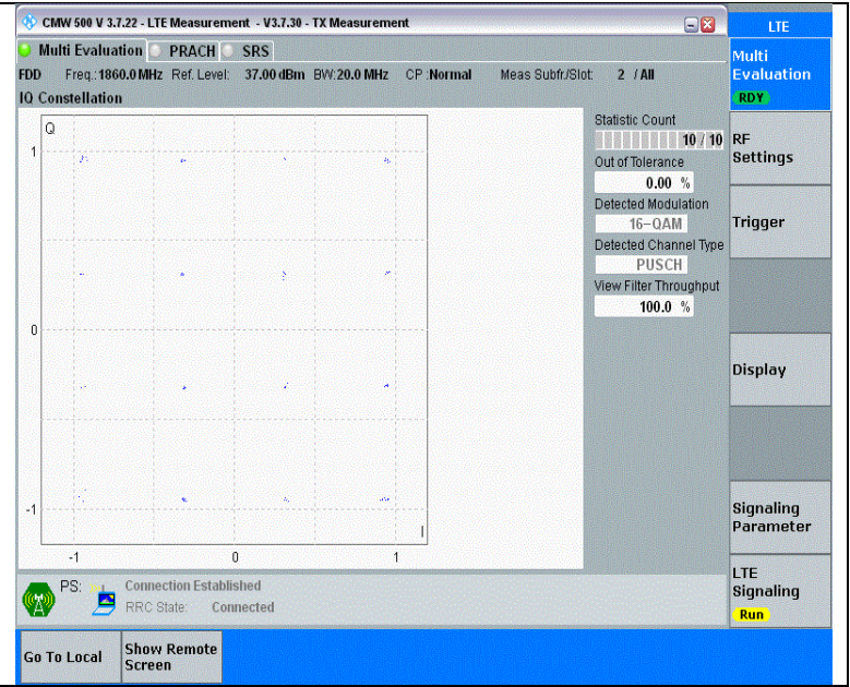
Band2-20MHz-16QAM-18700-1RB#0-PASS
