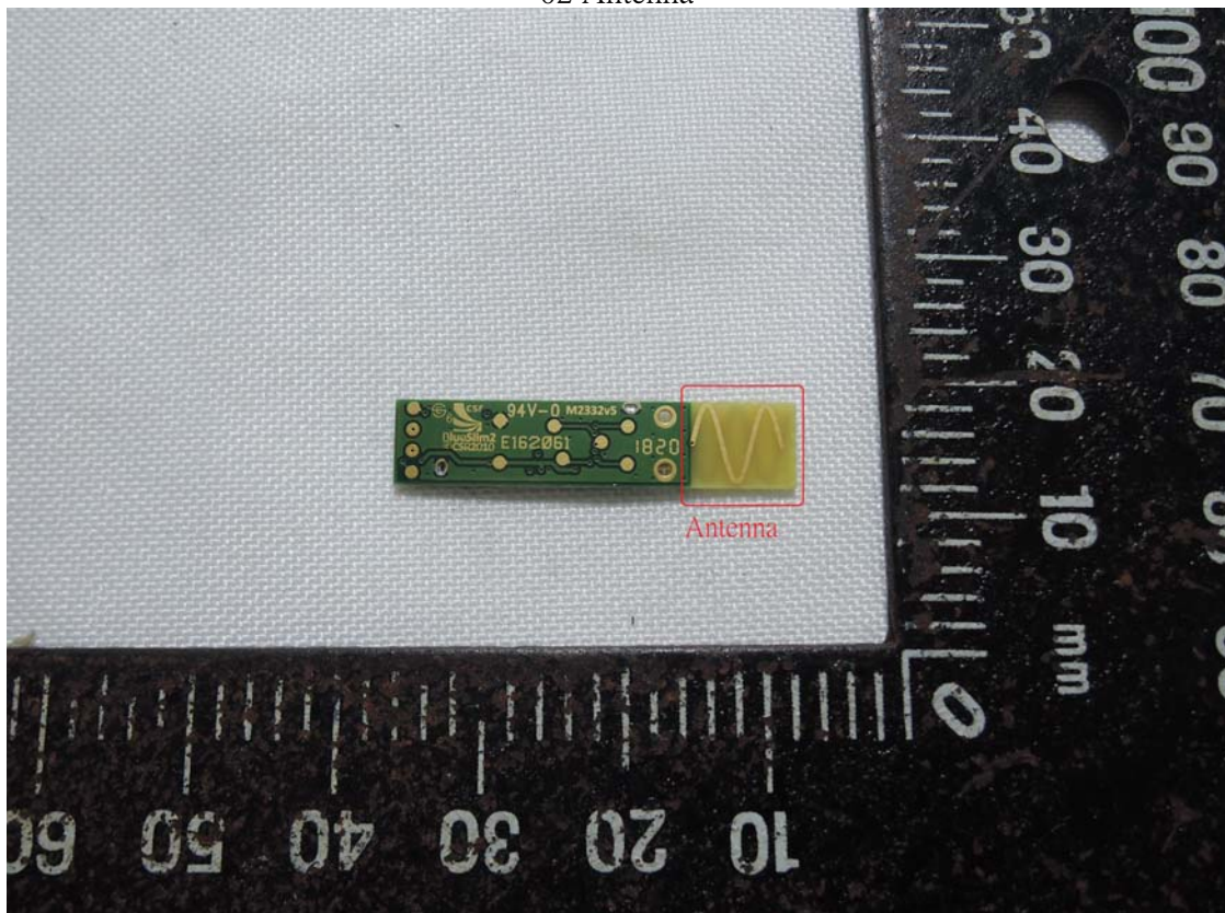
02 Antenna
