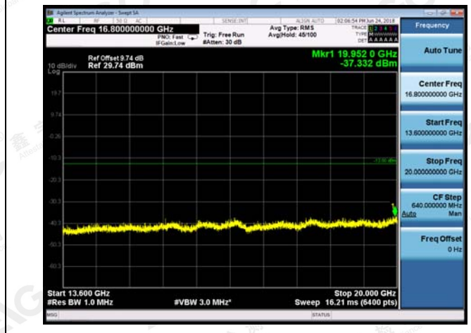
WCDMA 1700-MCH
