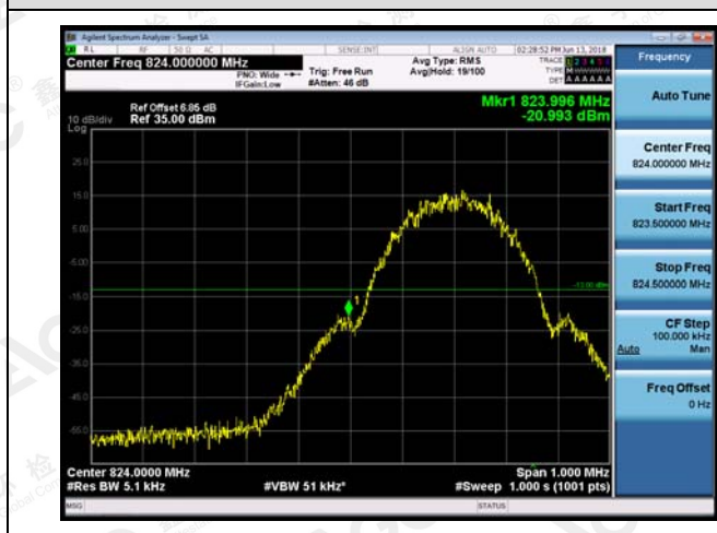
GSM 850-LCH-GSM
