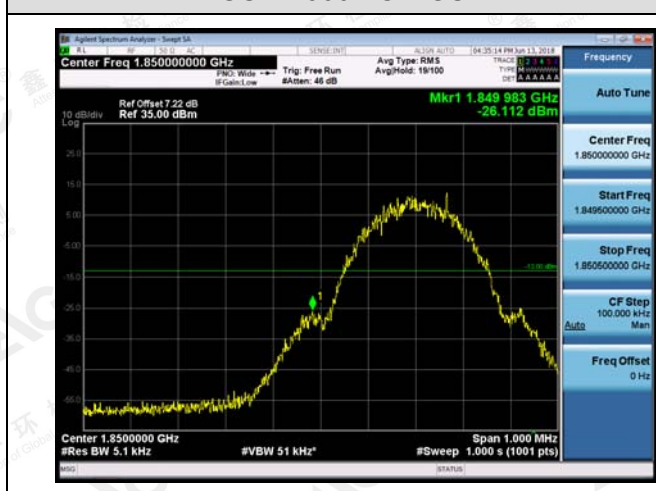
GSM 1900-LCH-GSM
