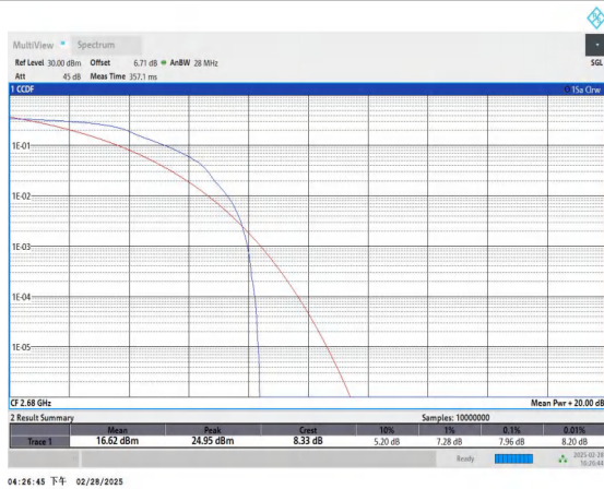
Band41-20MHz-QPSK-41490-1RB#0-PASS
