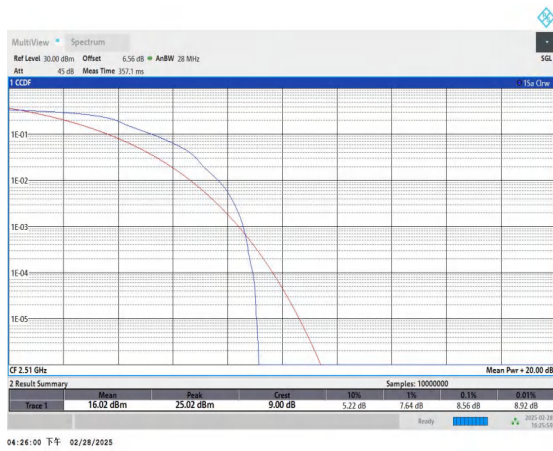
Band41-20MHz-QPSK-39790-1RB#0-PASS
