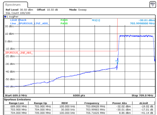
5MHz_Low_QPSK_25@0
