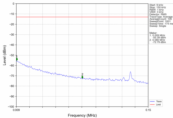
Band71_5MHz_QPSK_LCH_665.5MHz_RB_1_0_NTNV
