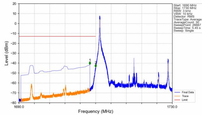
Band4_20MHz_QPSK_LCH_1720MHz_RB_1_0_NTNV
