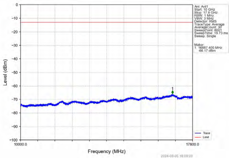
Band66_20MHz_QPSK_HCH_1770MHz_RB_1_0_NTNV
