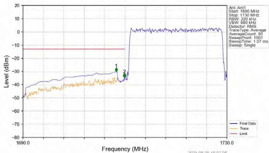
Band66_20MHz_16QAM_LCH_1720MHz_RB_100_0_NTNV
