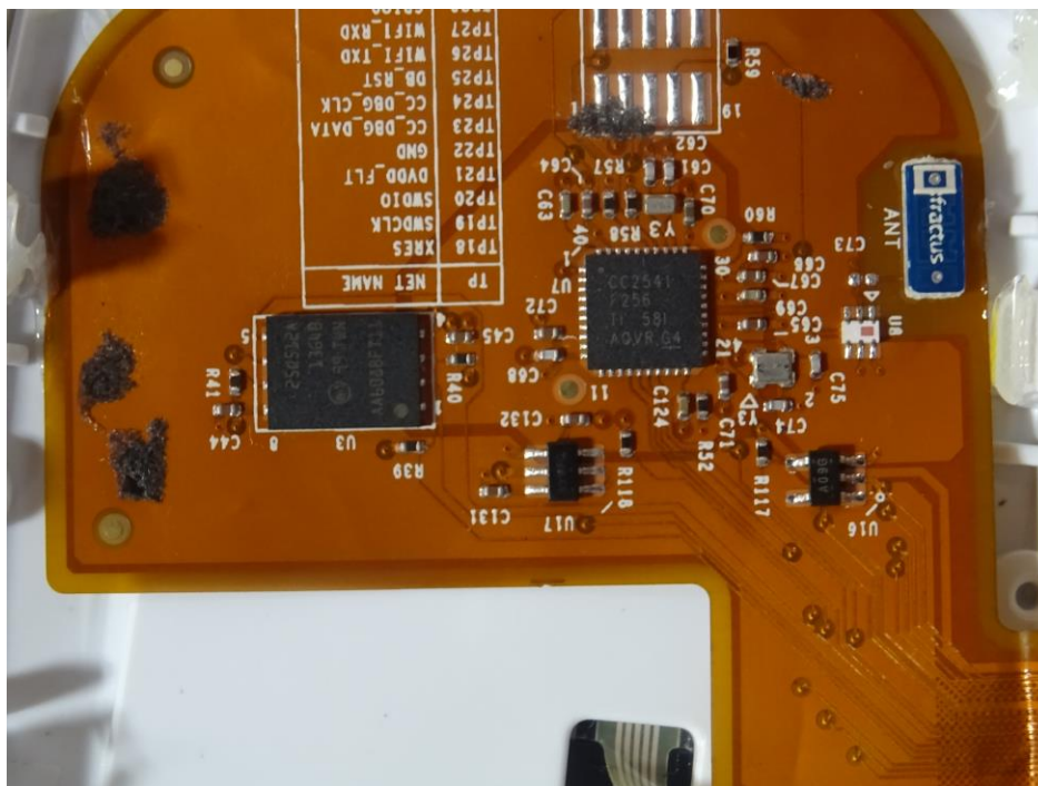
BLE chip and Antenna
