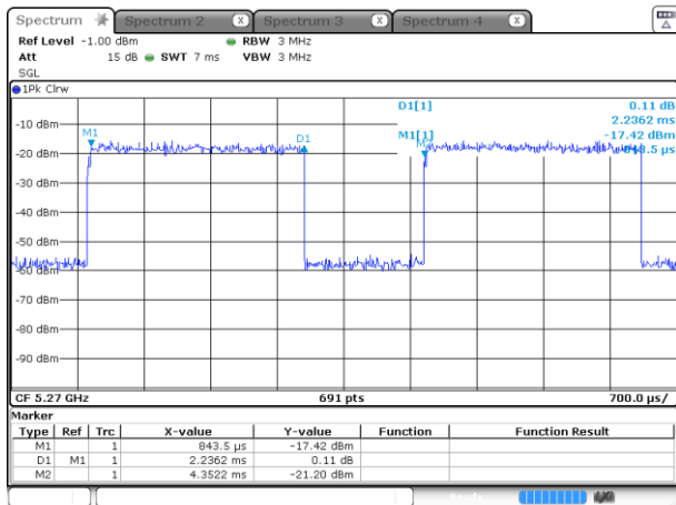
11n(HT40)-5270 MHz
