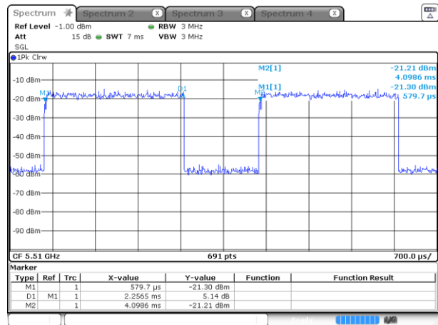
11n(HT40)-5510 MHz
