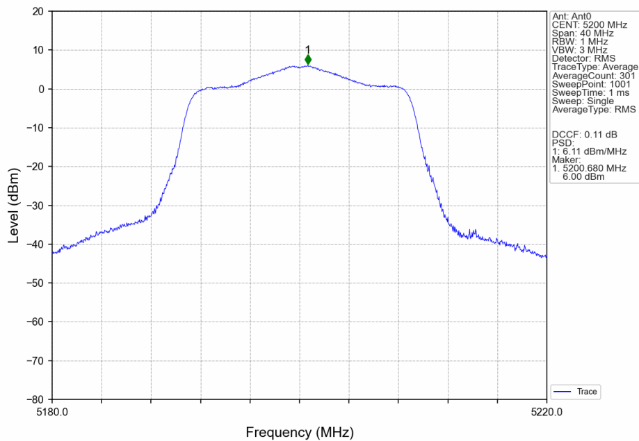
802.11n(HT20)_MCH_5200MHz_Ant0_NTNV
