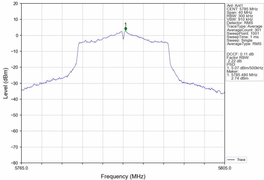
802.11n(HT20)_MCH_5785MHz_MIMO_NTNV
