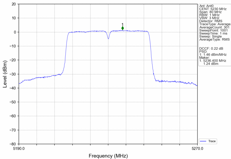
802.11ax(HEW40)_HCH_5230MHz_SU_Ant0_NTNV
