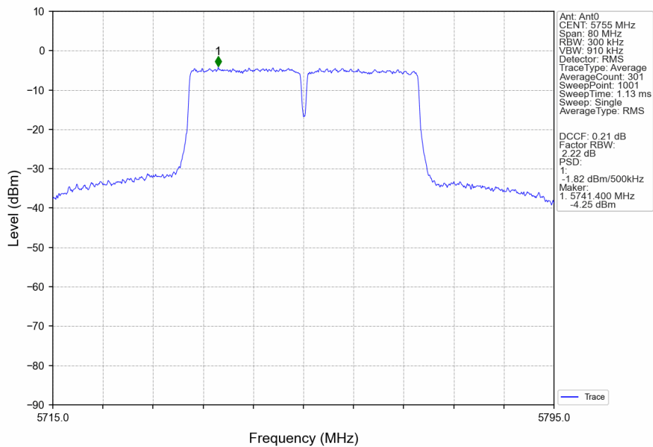
802.11n(HT40)_LCH_5755MHz_Ant0_NTNV
