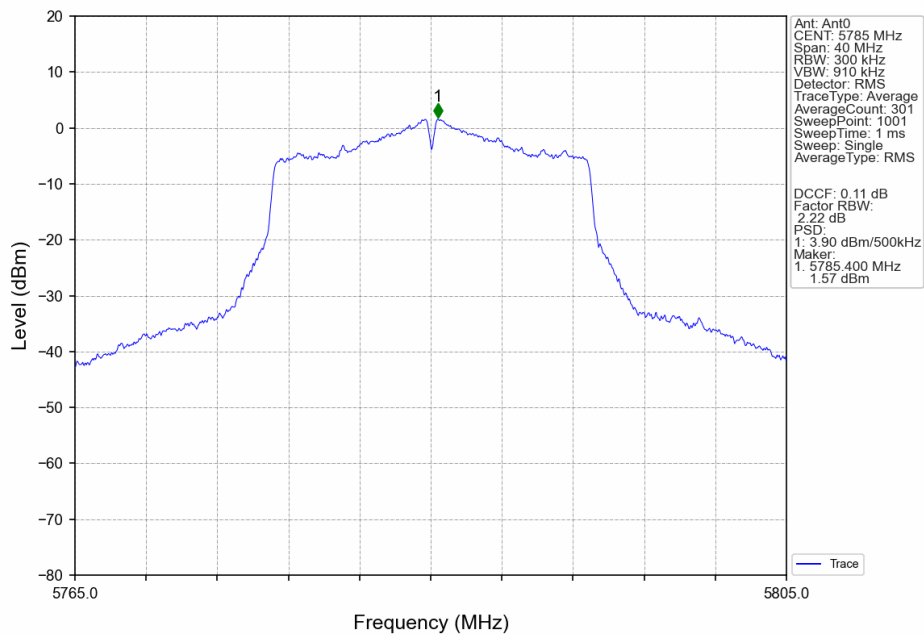
802.11n(HT20)_MCH_5785MHz_Ant0_NTNV
