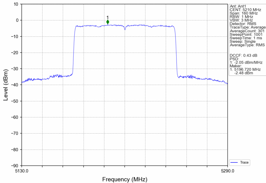
802.11ax(HEW80)_MCH_5210MHz_SU_Ant1_NTNV
