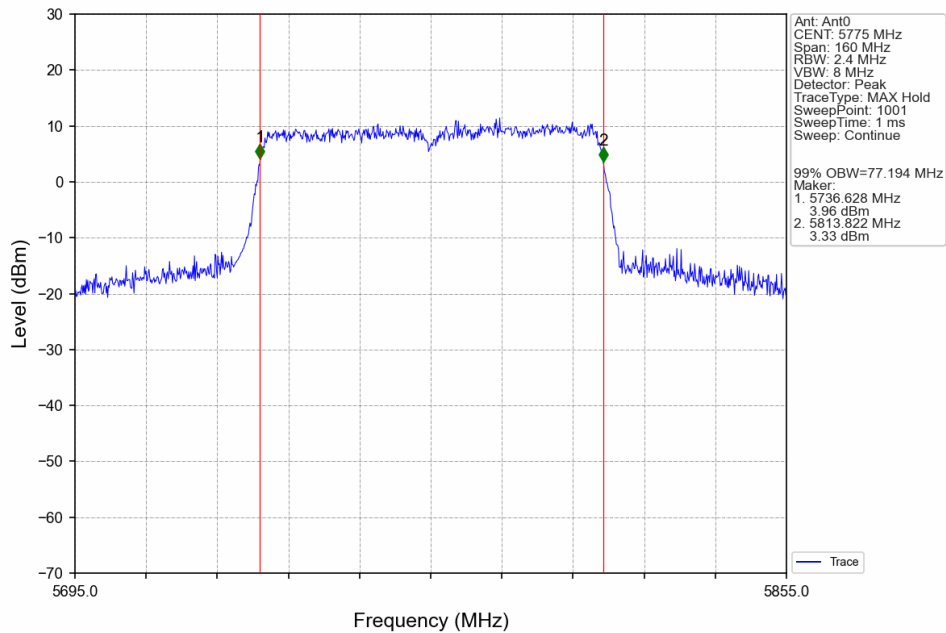
802.11ac(VHT80)_MCH_5775MHz_Ant0_NTNV
