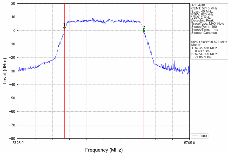
802.11ac(VHT20)_LCH_5745MHz_Ant0_NTNV
