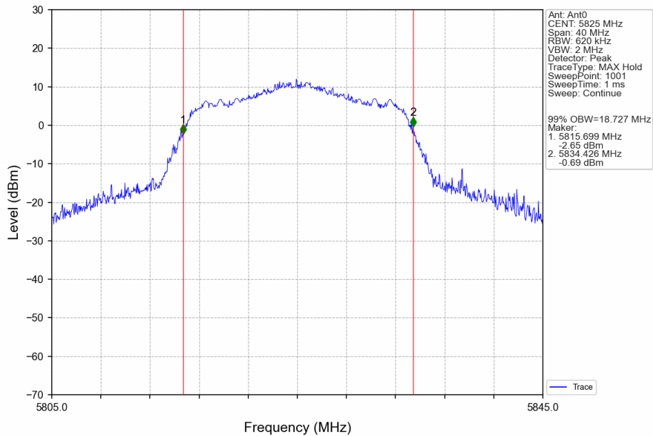
802.11n(HT20)_HCH_5825MHz_Ant0_NTNV
