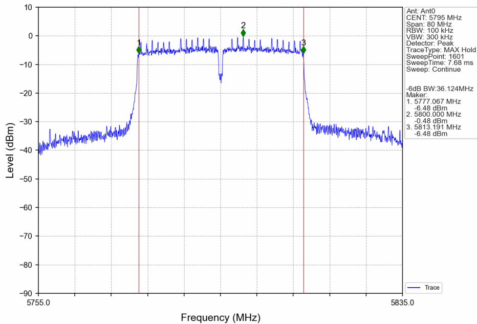
802.11n(HT40)_HCH_5795MHz_Ant0_NTNV
