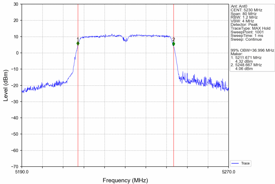
802.11ax(HEW40)_HCH_5230MHz_SU_Ant0_NTNV
