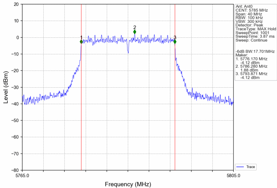
802.11ac(VHT20)_MCH_5785MHz_Ant0_NTNV
