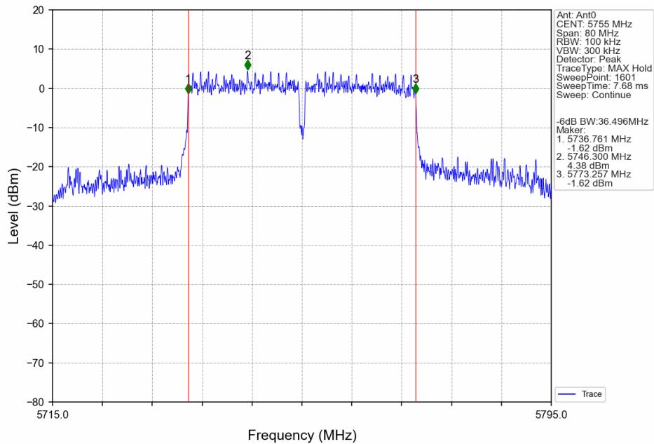
802.11ac(VHT40)_LCH_5755MHz_Ant0_NTNV
