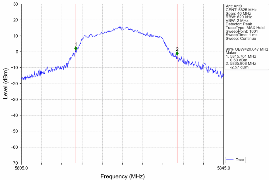
802.11a_HCH_5825MHz_Ant0_NTNV
