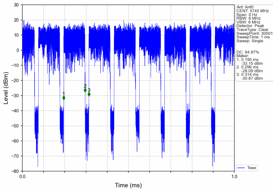
802.11ac(VHT20)_LCH_5745MHz_Ant0_NTNV
