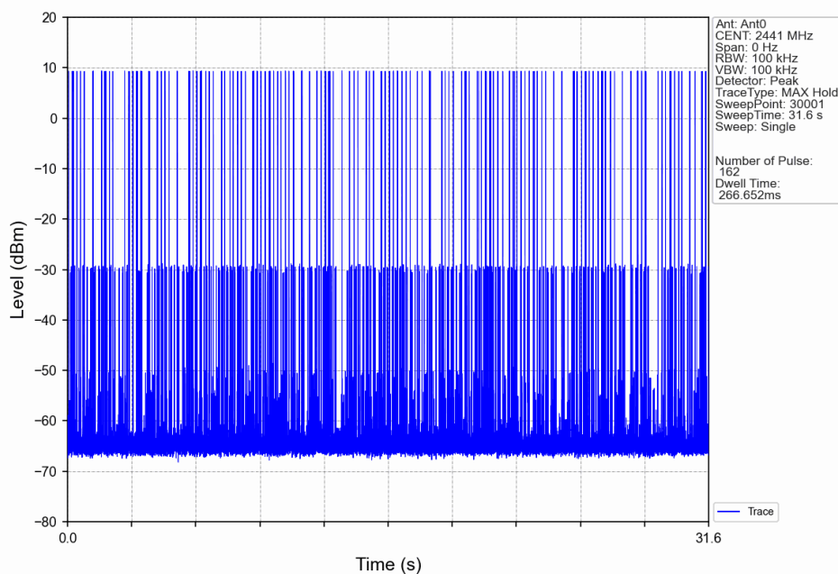
GFSK_DH3_HOPP_Ant0_NTNV
