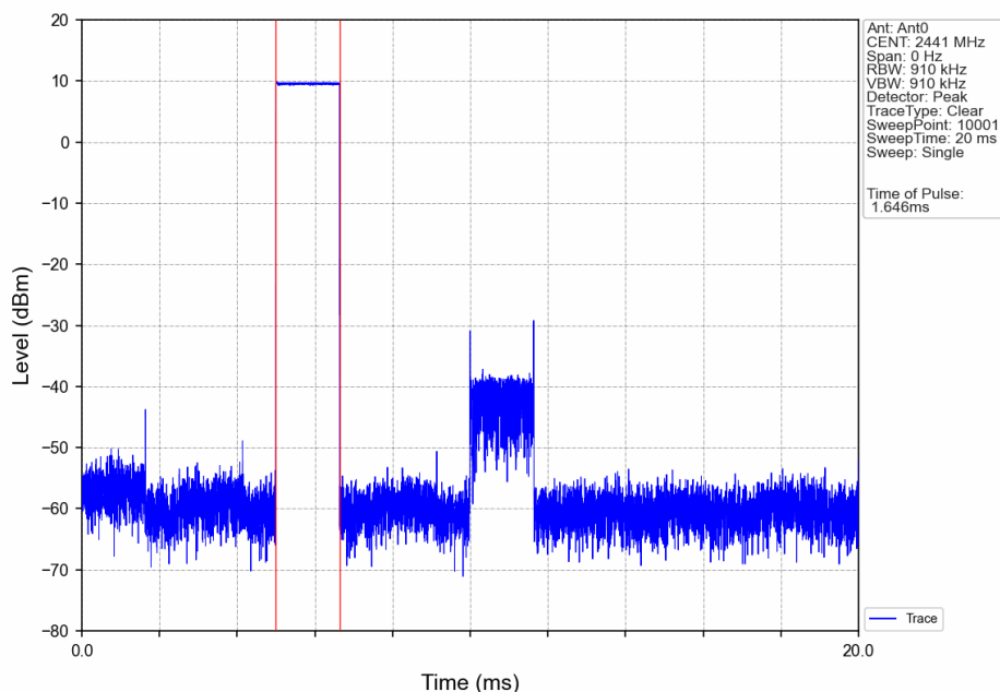
GFSK_DH3_HOPP_Ant0_NTNV
