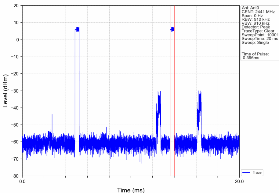
Pi/4DQPSK_2DH1_HOPP_Ant0_NTNV
