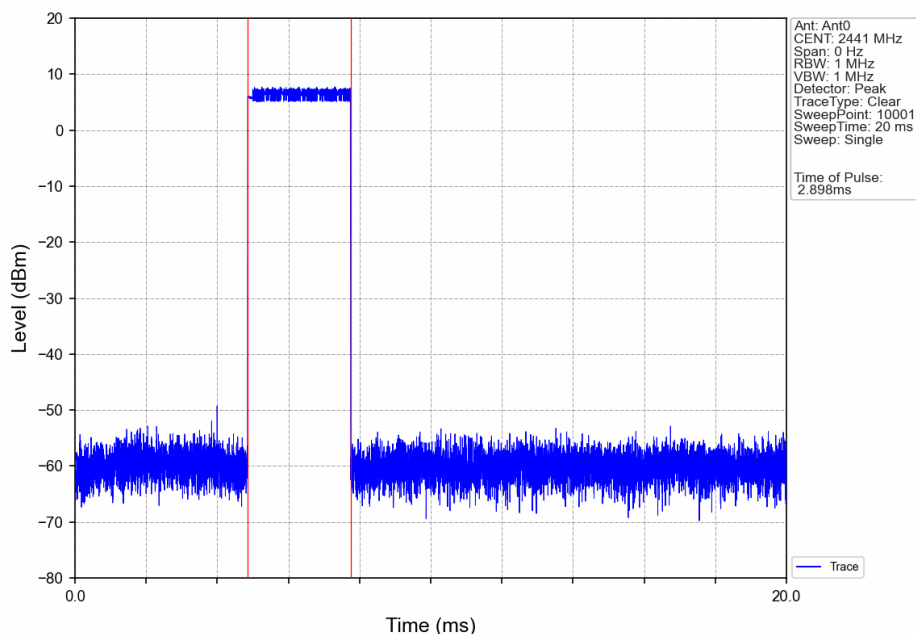
Pi/4DQPSK_2DH5_HOPP_Ant0_NTNV
