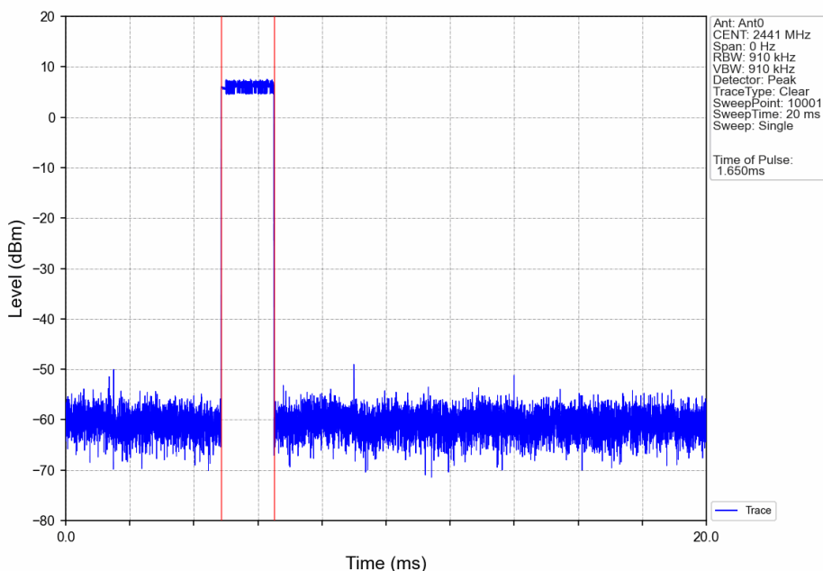
Pi/4DQPSK_2DH3_HOPP_Ant0_NTNV
