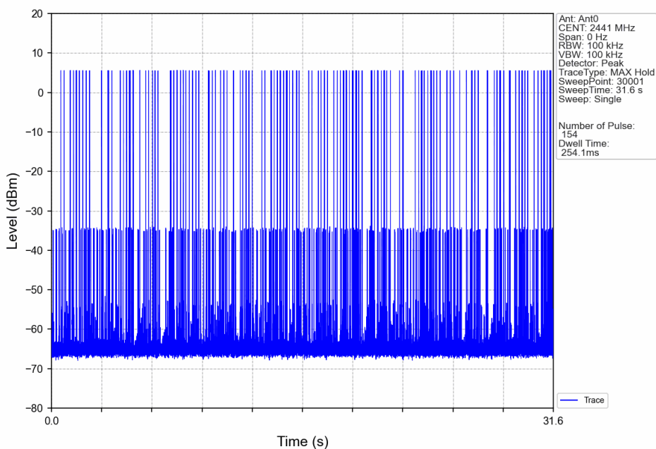
Pi/4DQPSK_2DH3_HOPP_Ant0_NTNV
