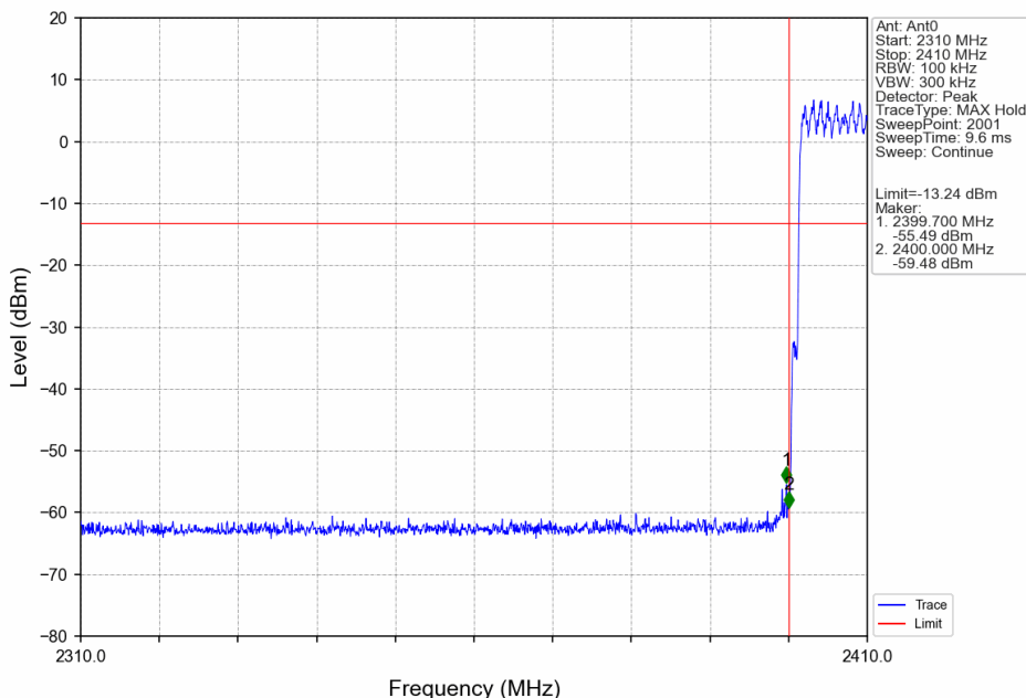
Pi/4DQPSK_2DH5_HOPP_Ant0_NTNV
