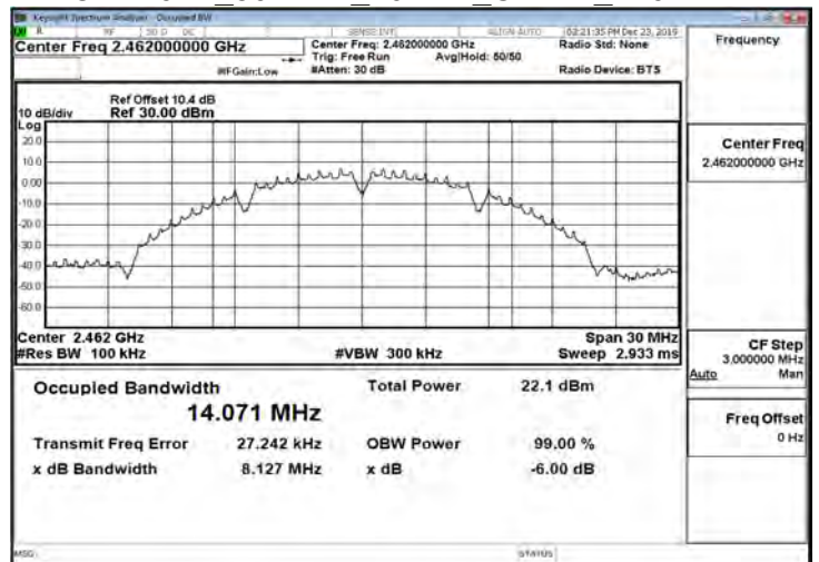
OBW 6dB 802.11b 20MHz Chain1 2462MHz
