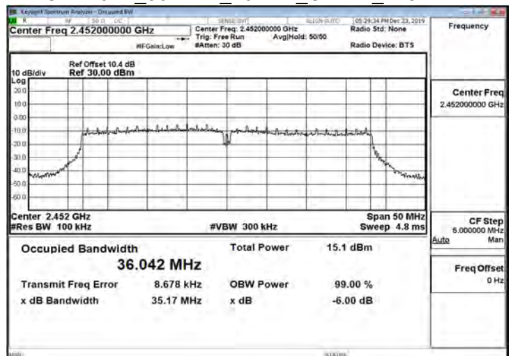
OBW 6dB 802.11n 40MHz Chain1 2452MHz
